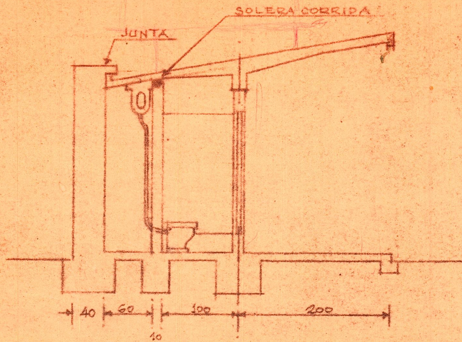
Sección
