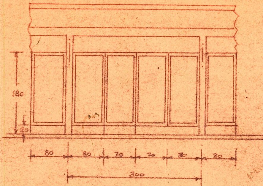
Fronte
