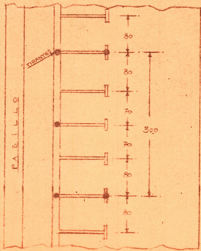
Planta
