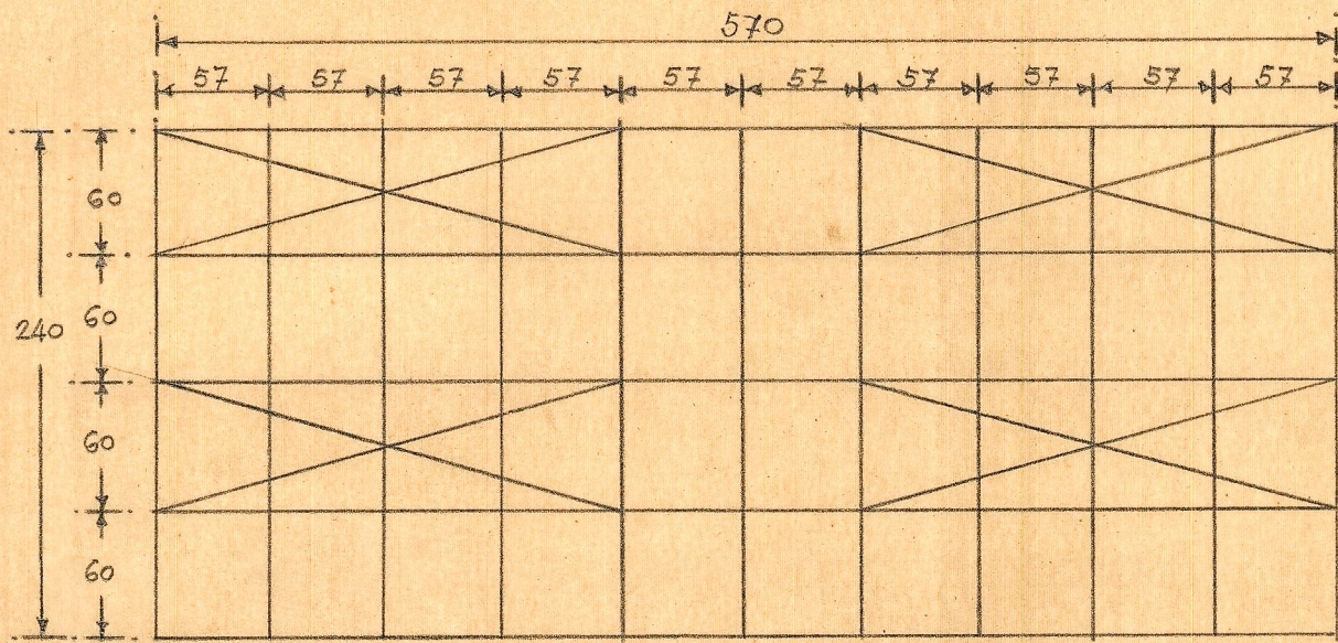
Vidrieras de las plantas altas o bajas ESCALA = 1:40
