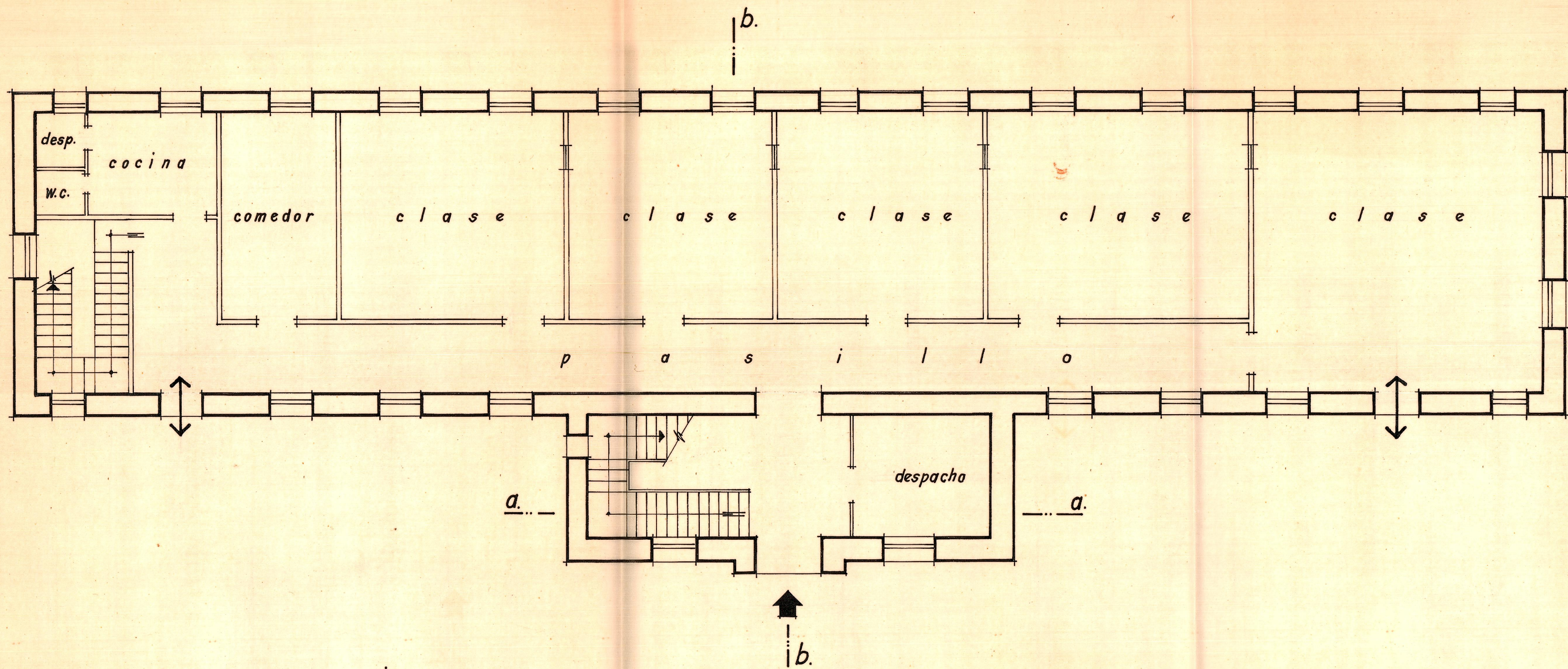
planta baja
