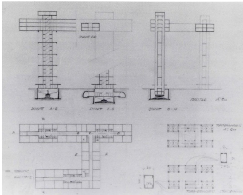
f.A9. El Lissitzky. Vistas (1924/1925) 37,2 x 46,0 cm
