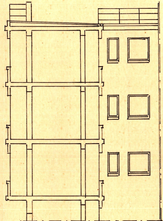
SECCION A-B
