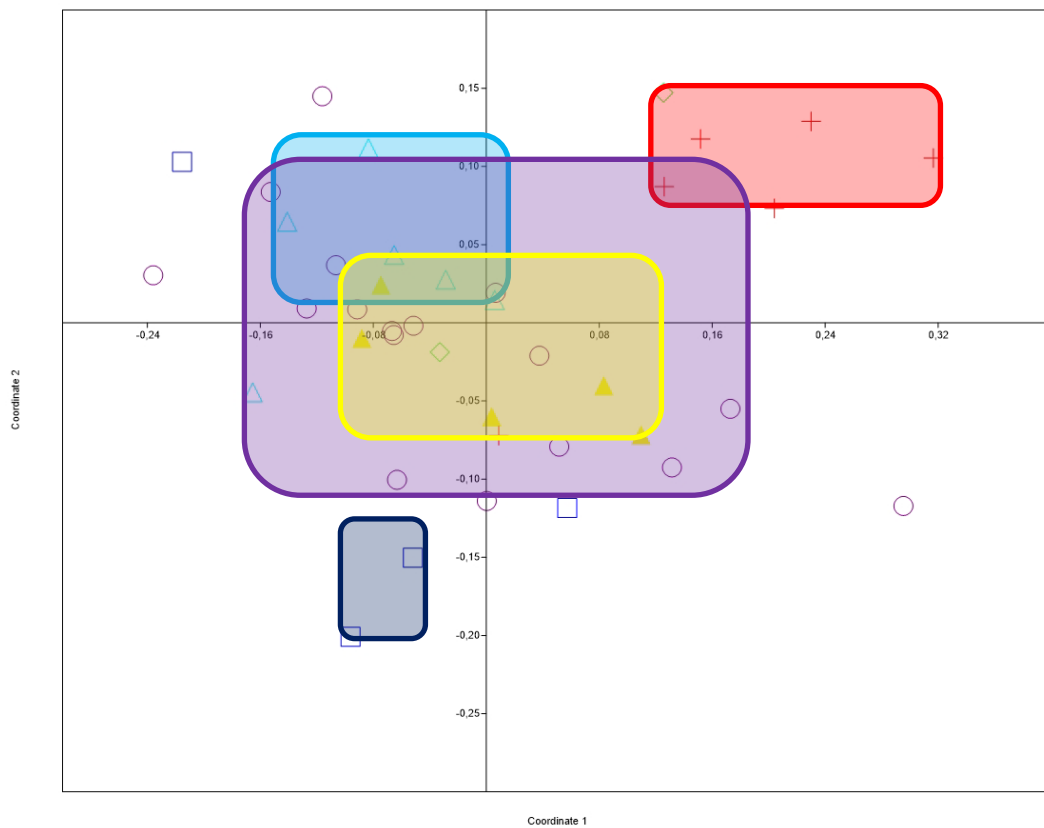
Fig. 3.10b MDS Box Color -Dental Metrcs
