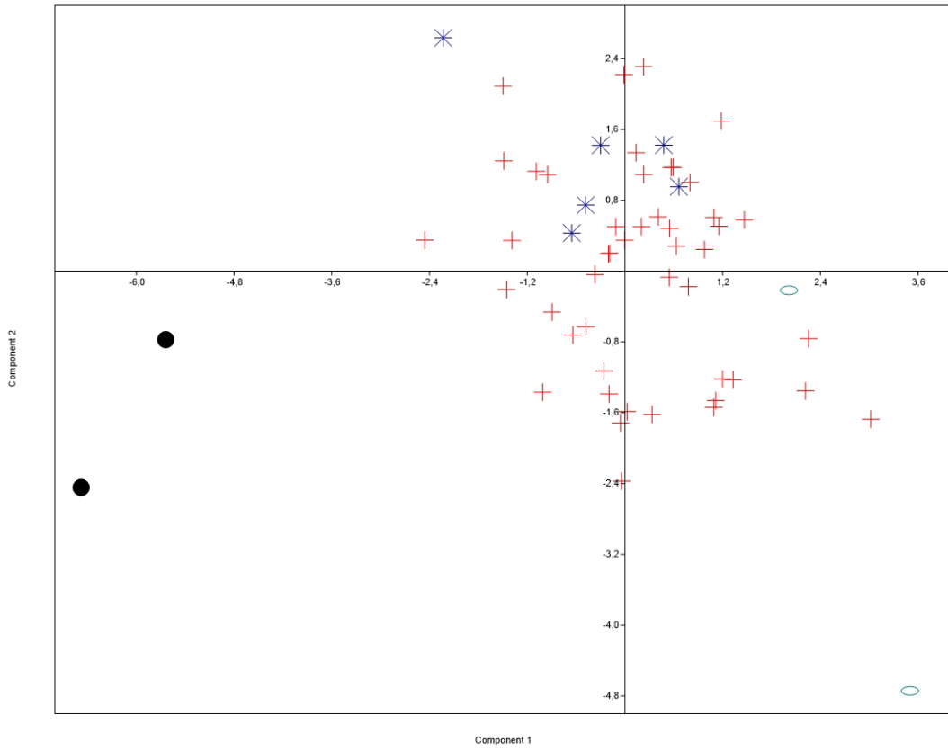
Fig. 3.30a PC1vsPC3
