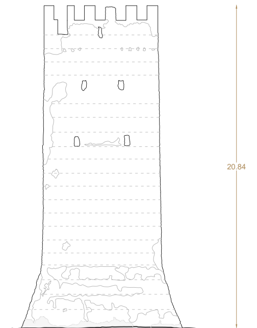
ALÇAT
