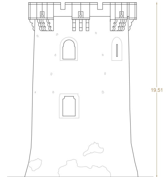
ALÇAT
