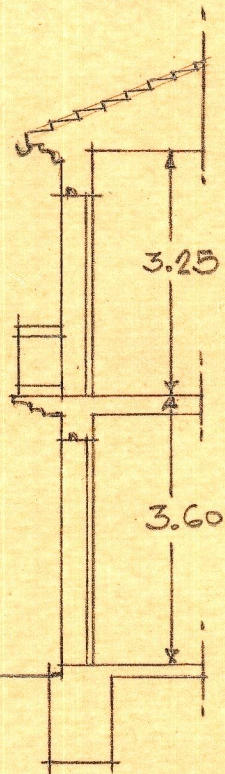
Sección
