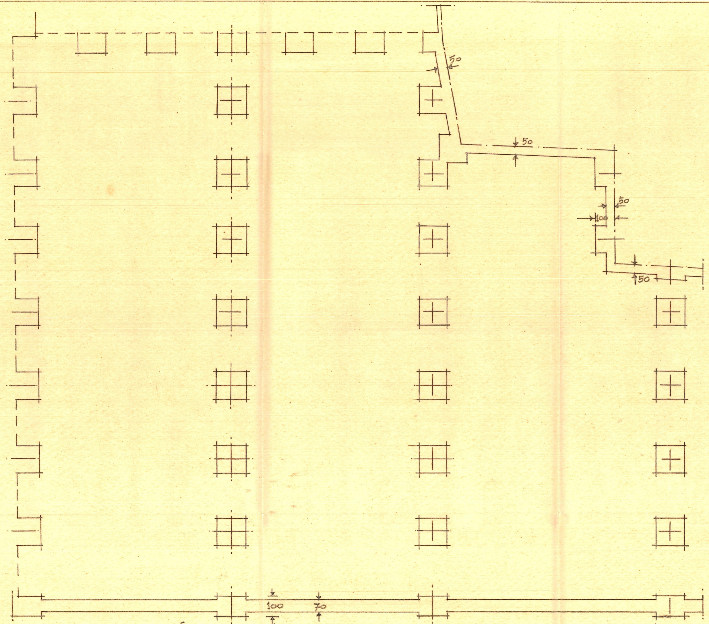
Planta de Cimentación de los pilares de 1.50x1.50
