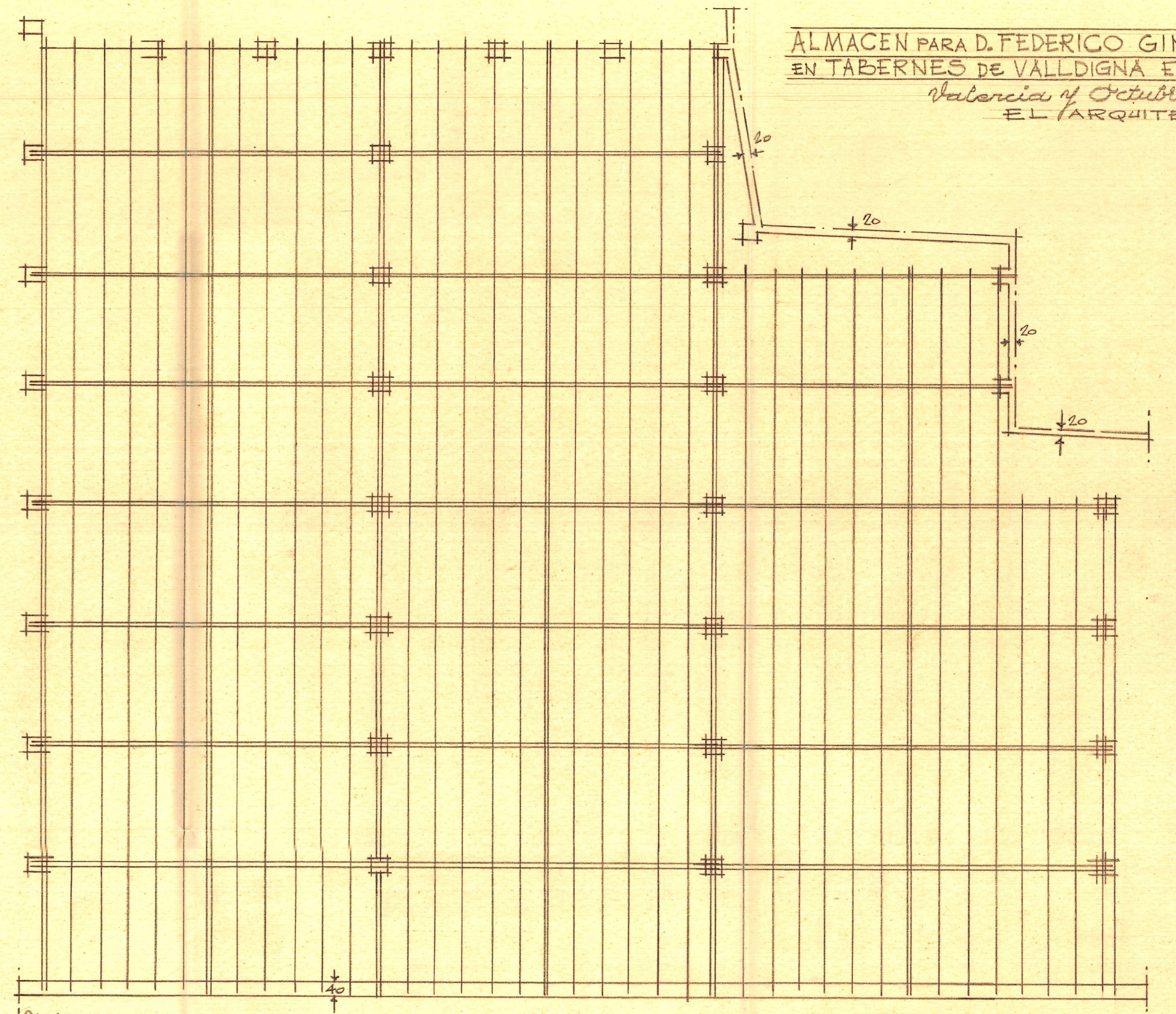
Subramado de cubierta = Pilares de 0.50x0.50 Armaduras de perfiles laminados Viguetas madera de 20x7 cubierta de fibrocemento
