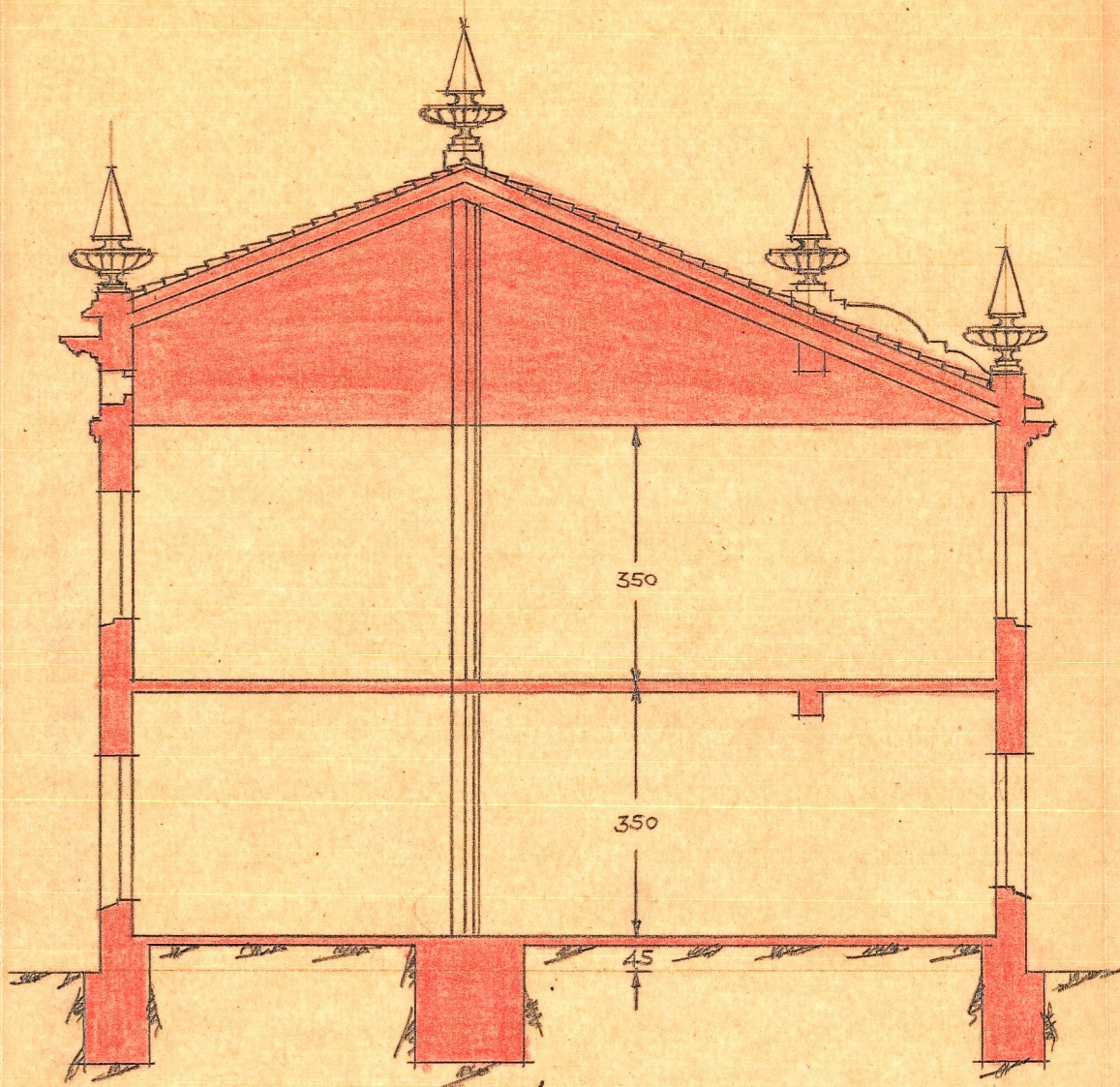
Sección por AB
