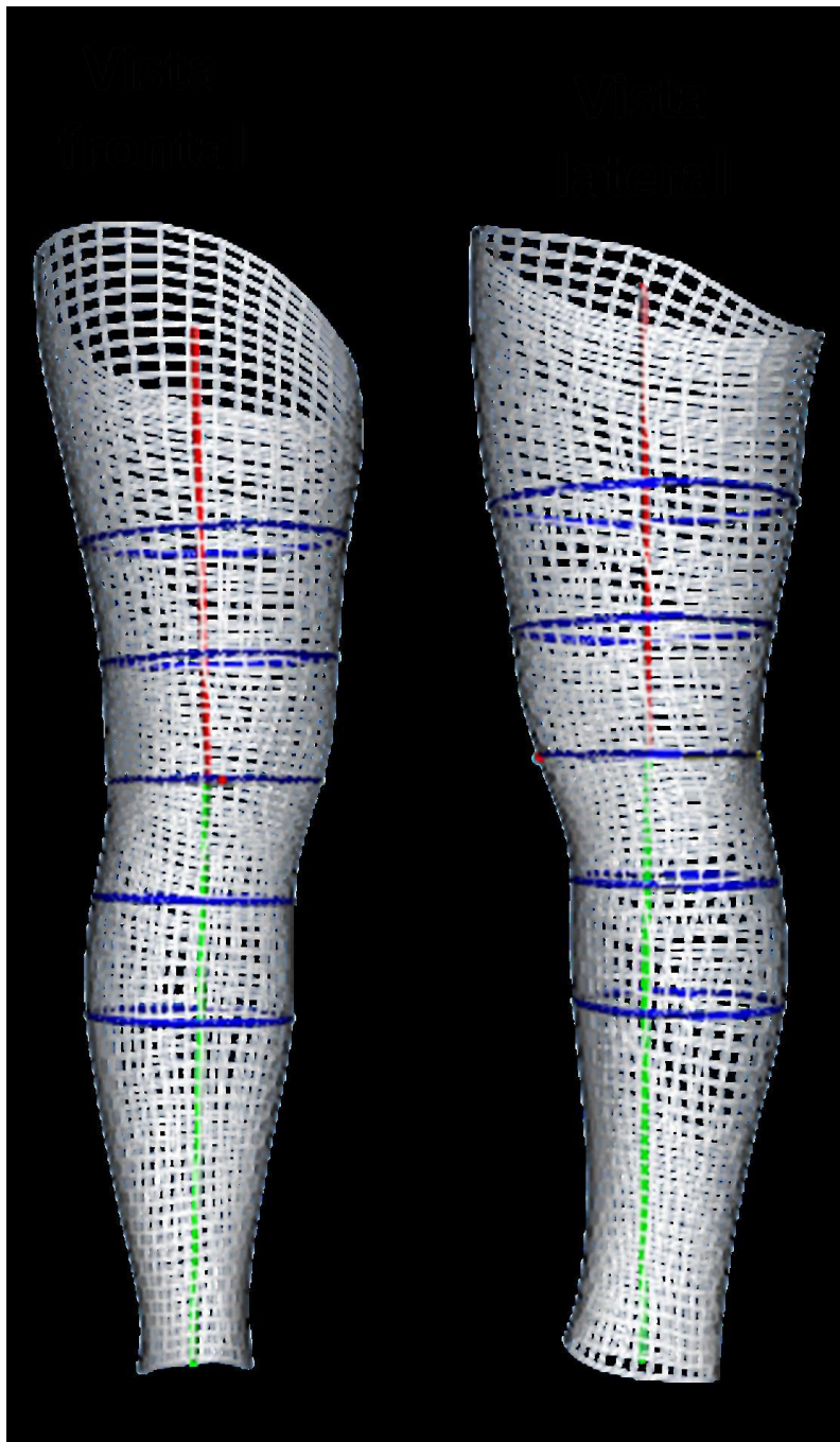
Figura 9.- Morfotipo de pierna para su uso como patrón de diseño de la ortesis de la talla L.
