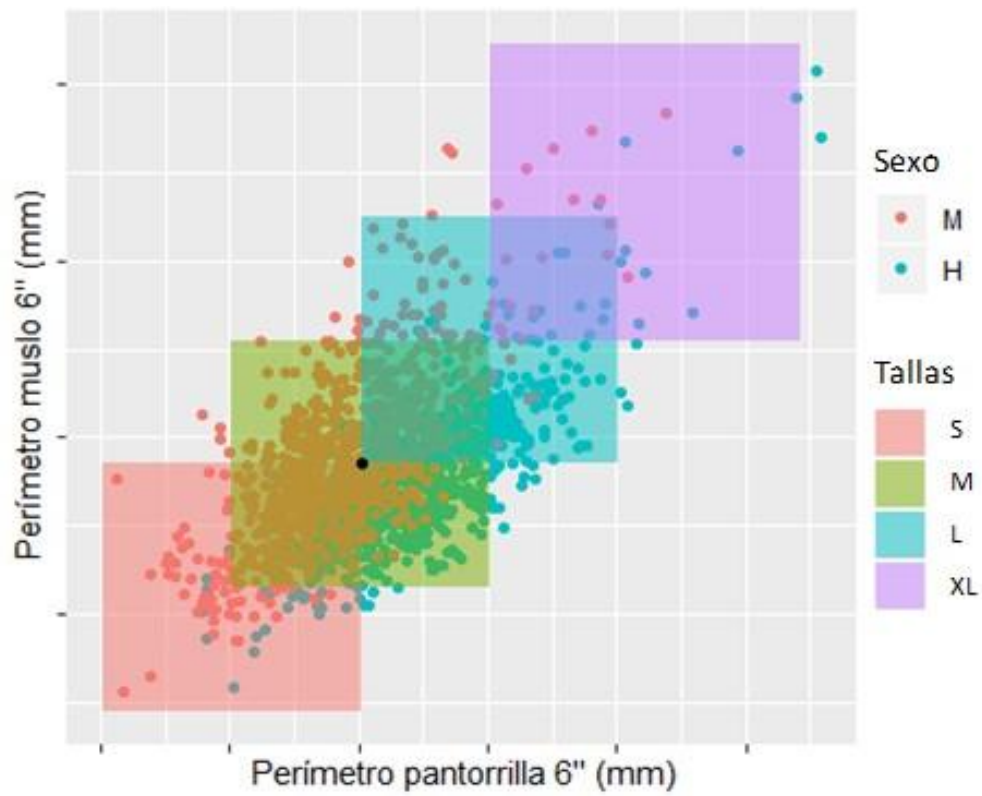
Figura 8.- Propuesta de tallaje de la ortesis de rodilla en base a 4 tallas cubriendo el 93% de la población objetivo.
