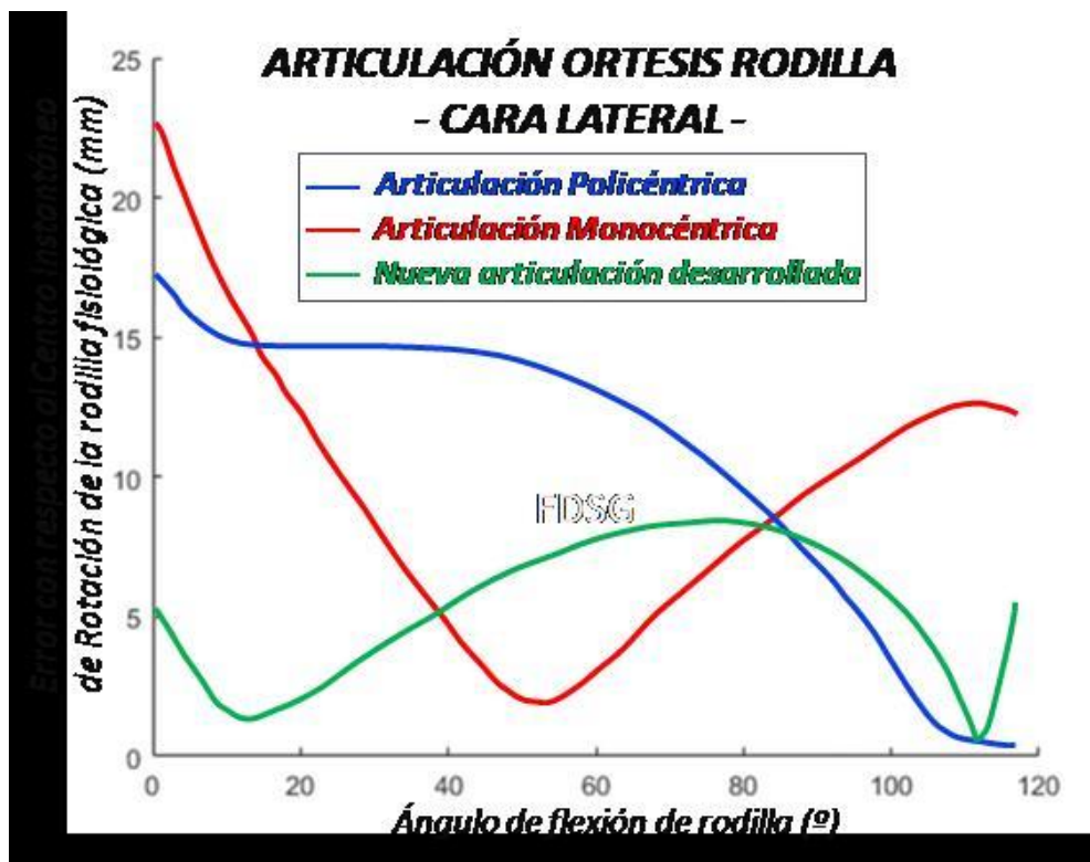
Figura 7.- Error cometido de la nueva articulación desarrollada (cara lateral) con respecto al Centro Instantáneo de Rotación de la rodilla fisiológica. Comparación con el error cometido por otras articulaciones disponibles actualmente en el mercado (mono- y policéntricas).
