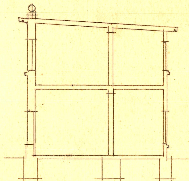
Seccion por A-B.
