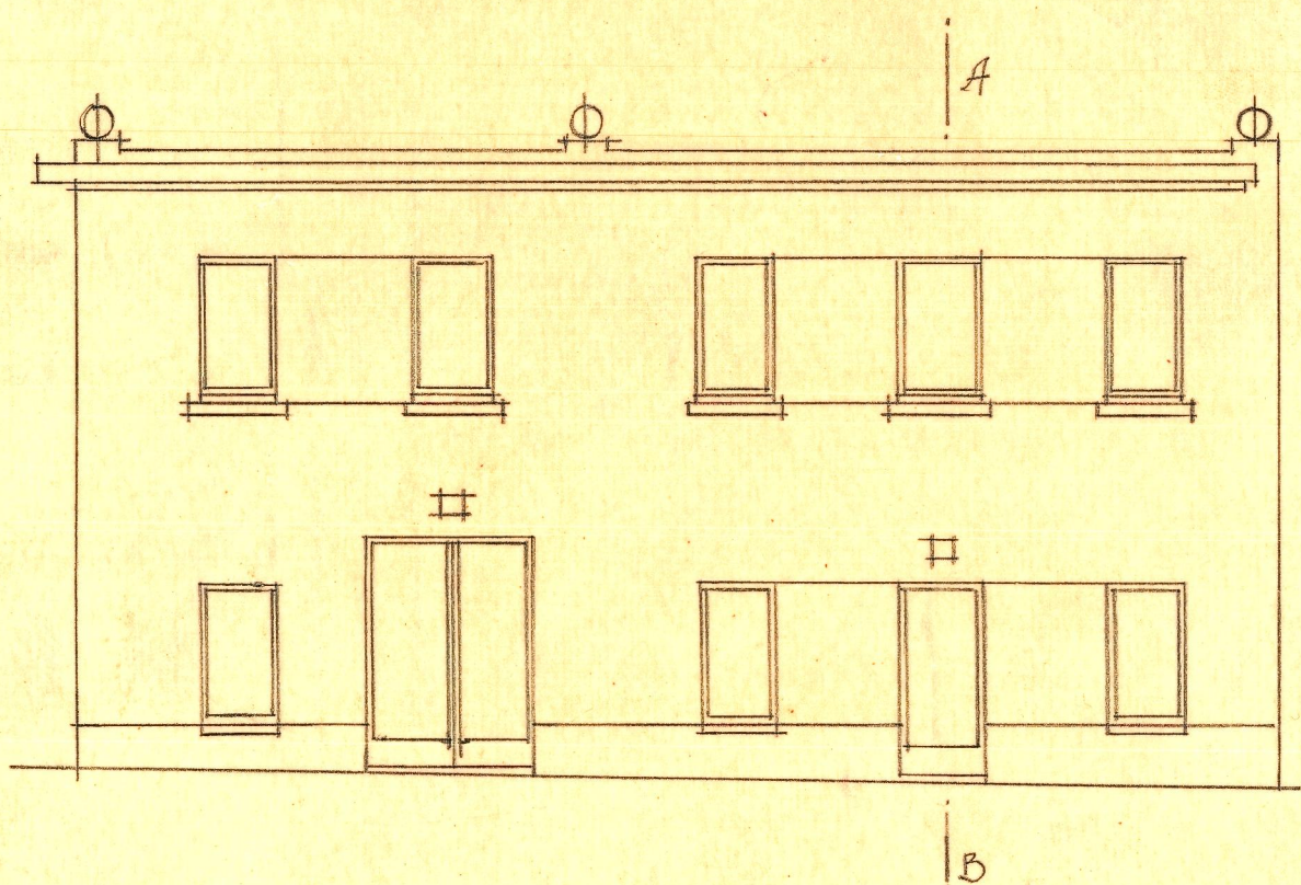
Fachada a la Calle de Padilla
