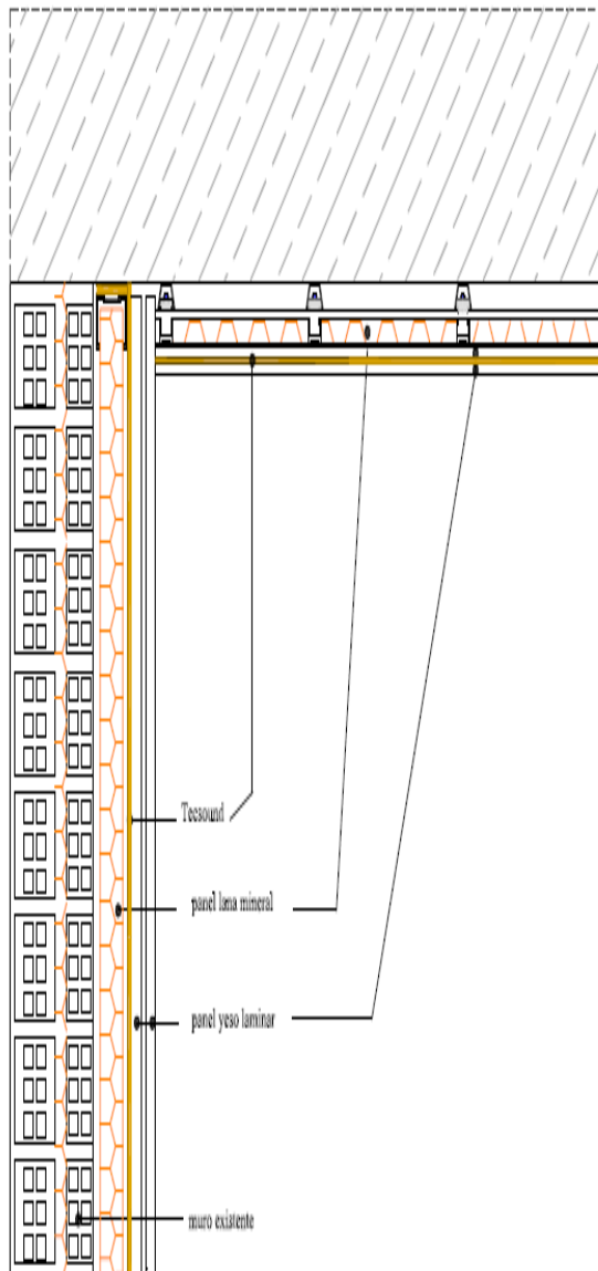
ENCUENTRO TECHO CON MEDIANERA
