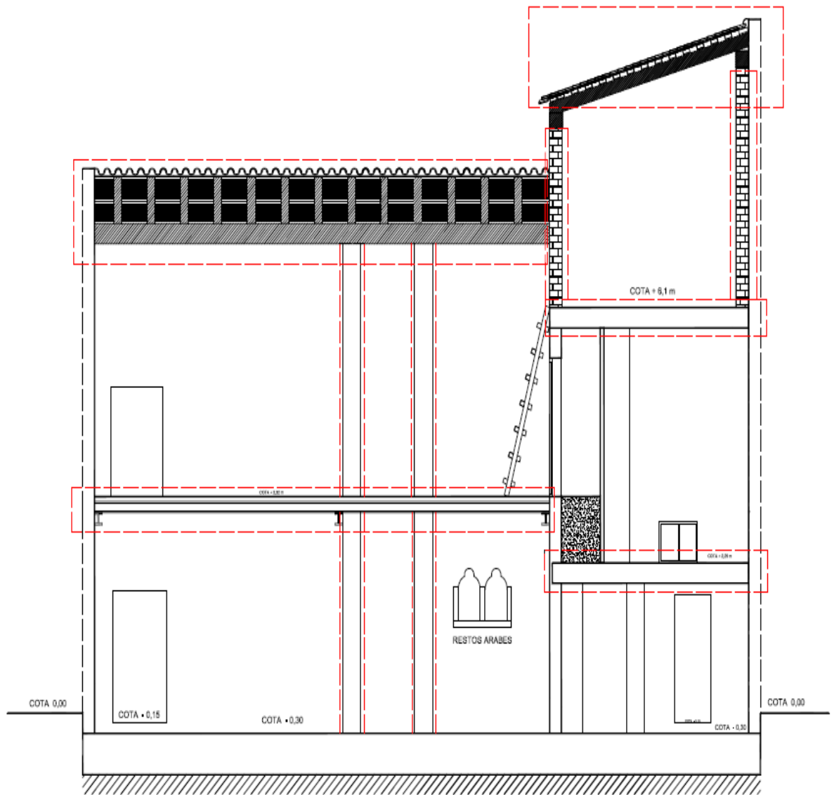
Sección con las patologías remarcadas de aquellas zonas que precisan intervención
