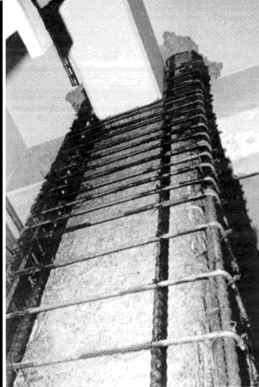
SOPORTE RECRECIDO HORMIGÓN
