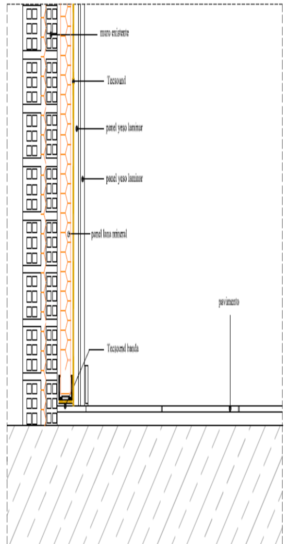
ENCUENTRO MEDIANERA CON PAVIMENTO
