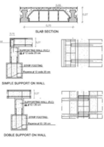
Sanitary Slab Forjado sanitario
