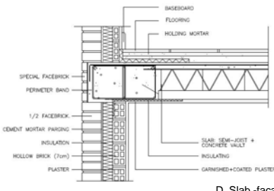
D. Slab -facade D. Fdo -fachada
