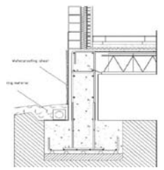
D. Slab -facade D. Fdo -fachada
