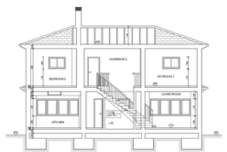
S.C-C'
