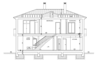
S. B-B'
