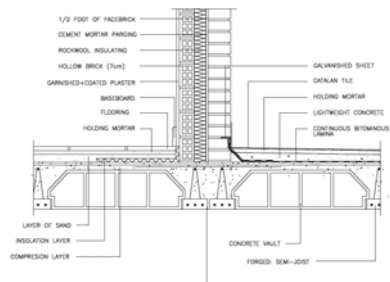
D. Slab -facade D. Forjado -fachada
