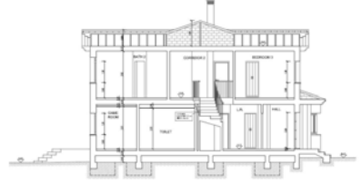
S. A-A'
