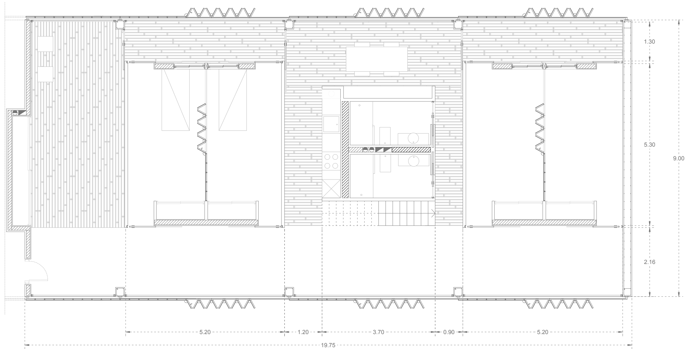
5.1.4. PLANTA TIPO Detalles en planta ESCALA 1:75 Instalaciones de tratamiento y depuración de aguas residuales y grises. Trabajo Final de Grado 2017/2018
