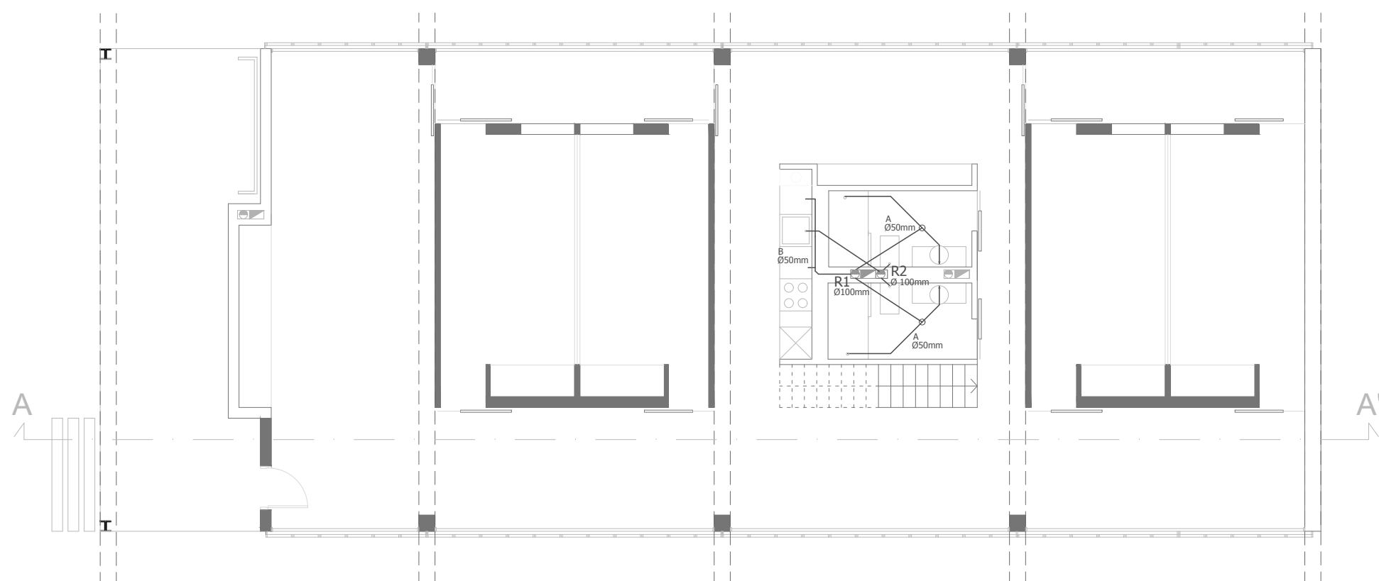
PLANTA SANEAMIENTO
