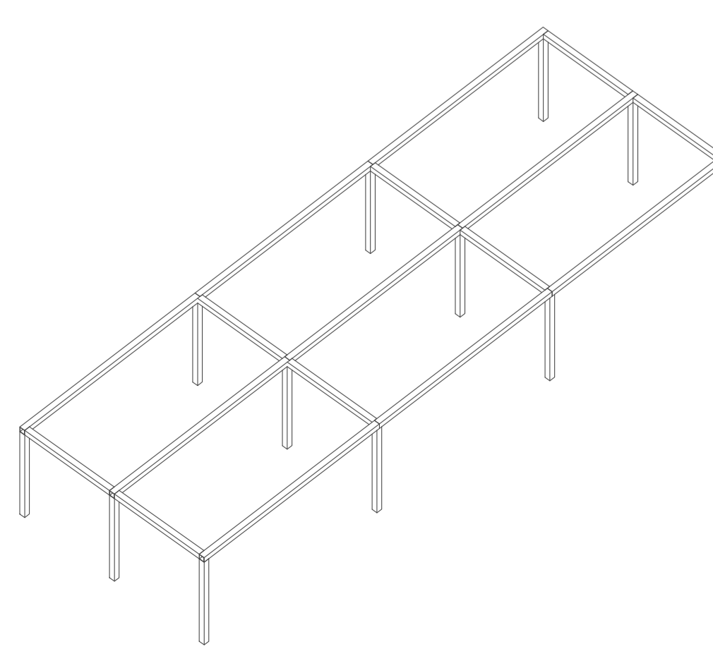
ESTRUCTURA SECUNDARIA
