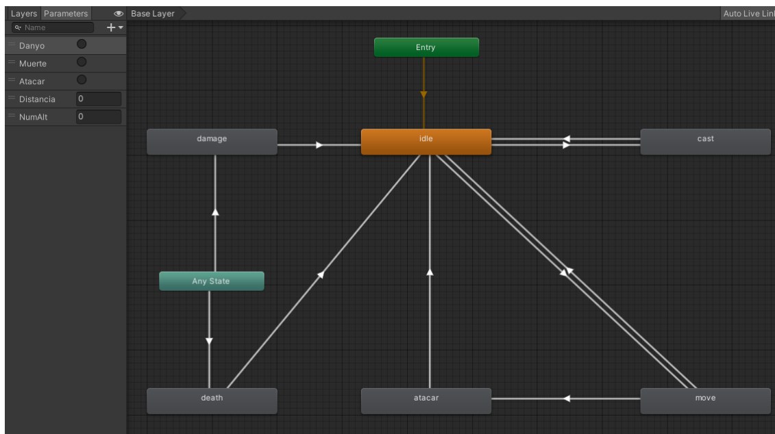
Imagen 35: Máquina de estados de los jefes
