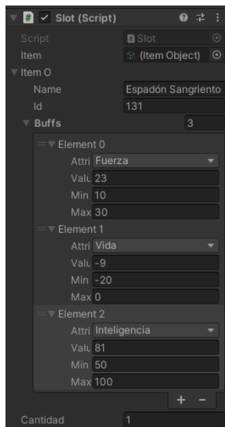
Imagen 38: Slot inventario con un ItemObject
