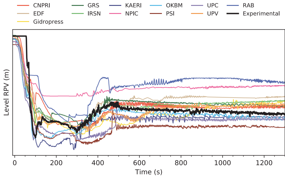
Fig. 20. RPV level.
