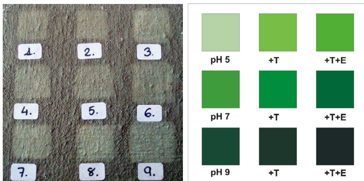
Figuras 2a y 2b - Influencia del pH, tensoactivo (T: 0,5ml de Tween® 20) y espesante (E: 2,5g de Tylose® MH 300P) en la efectividad del ácido cítrico (0,5g/50ml de agua destilada) salificado con TEA
