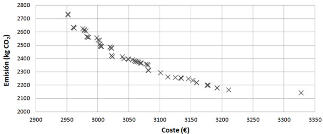
Figura 3. Coste frente emisión de CO 2 . Frontera de Pareto
