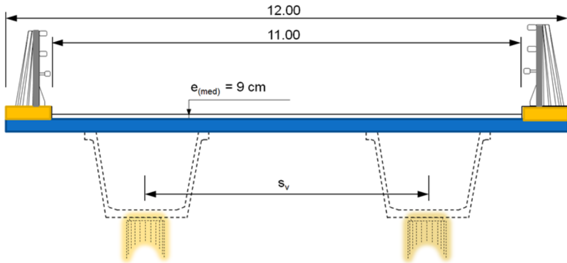
Figura 2. Sección transversal del puente
