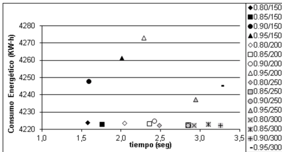
Figura 3 Consumos medios de las soluciones óptimas empleando el método SA.
