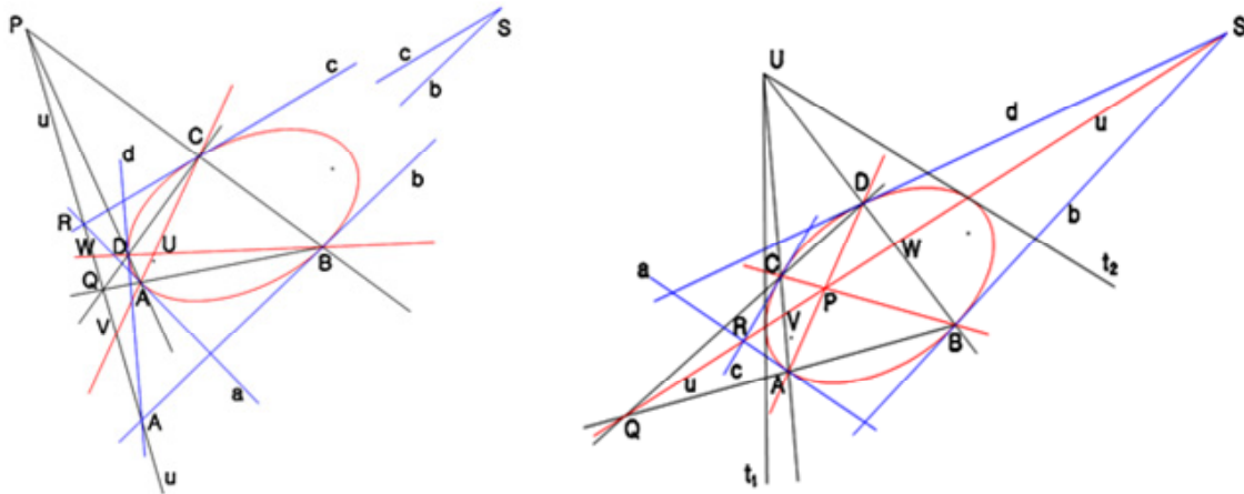
Figura 5. Representaciones de la construcción de la recta Polar de un punto respecto a una cónica. Cuando el punto ( U ) es interior a la cónica (en este caso una elipse) y cuando el punto ( U ) es exterior.
