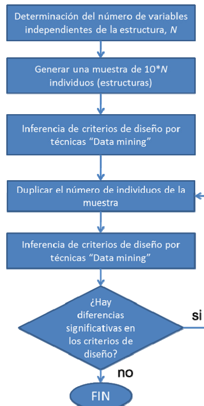
Figura 2 Flujo del procedimiento CGD para la generación de bases de datos de estructuras óptimas
