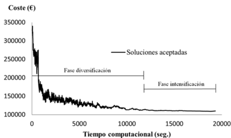
Figura 5. Evolución del coste respecto al tiempo para la mejor solución
