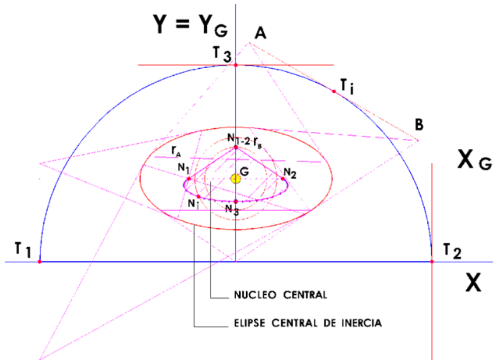
Figura 14. Cálculo del Núcleo Central de de la sección semicircular de radio 2cm. Los puntos del Núcleo han sido obtenidos mediante el cálculo de los Polos recíprocos, respecto a la Elipse Central de inercia calculada previamente, de las rectas tangentes al perímetro de la superficie. Cada recta tangente tiene un polo recíproco respecto a la elipse. Su simétrico respecto al C.D.G. (Centro de la Elipse), antipolo, es un punto del Núcleo Central.
