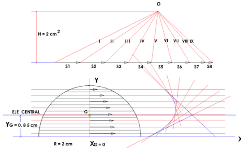
Figura 8. Determinación grafostática del Centro de Gravedad de la superficie de un semicírculo con centro en el origen de coordenadas y radio R = 2 cm.
