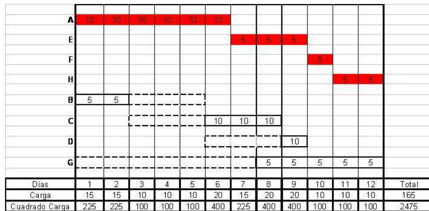
Figure 9: Calendario de ejecución y diagrama de cargas (2ª nivelación)
