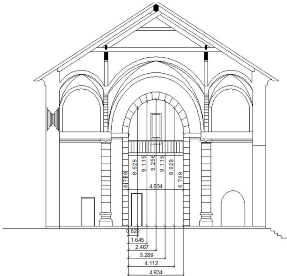
Figura 2: Sección con vistas al coro
