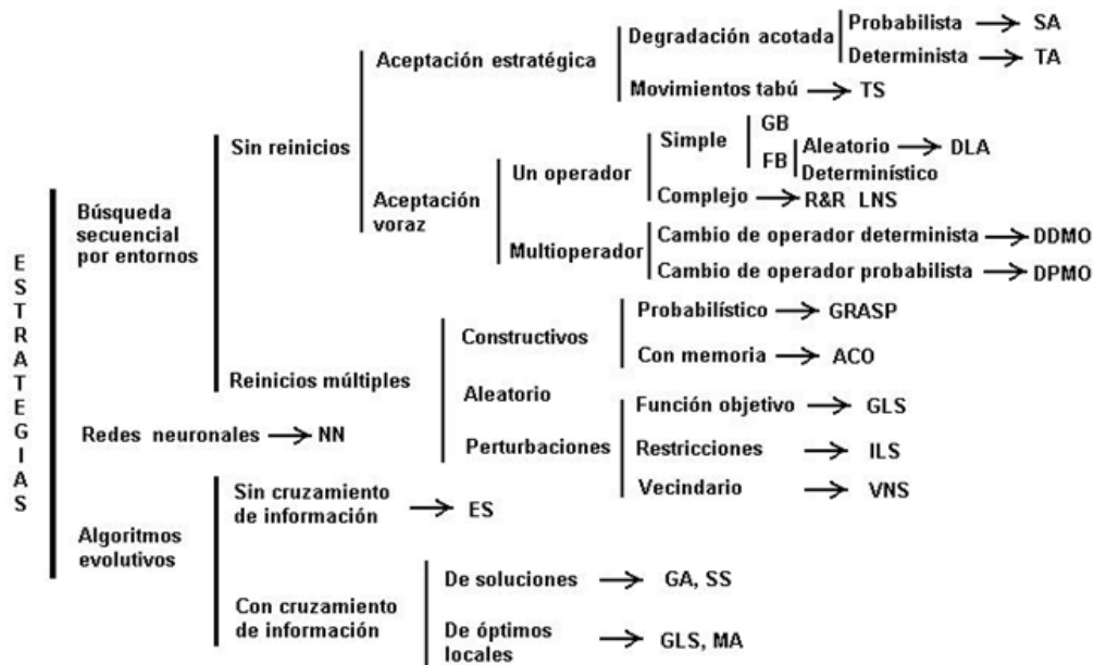
Figura 3 Taxonomía de estrategias empleadas en la resolución aproximada de problemas de optimización combinatoria (Yepes, 2002)
