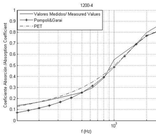
Figura 7 coeficiente de absorción en incidencia normal, comparación entre valores medidos y predichos por distintos modelos. Poliéster Reciclado 400 g/m 2 y 40 mm de espesor.
