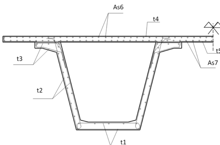
Figura 4. Variables de la armadura pasiva en losa y viga
