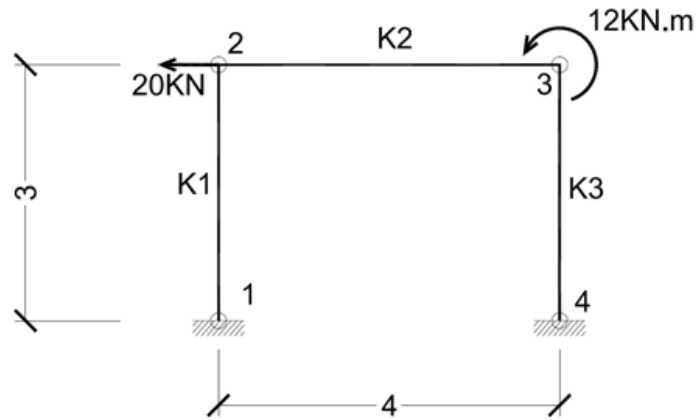
Figura 2: Croquis del pórtico a calcular
