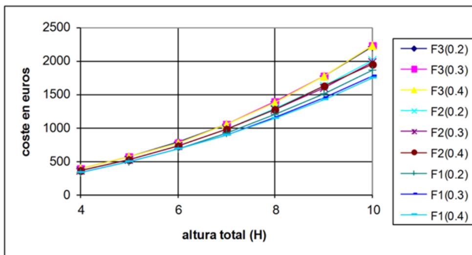
Figura 3 Relación entre la altura total del muro (H), en metros, y su coste por metro lineal en euros
