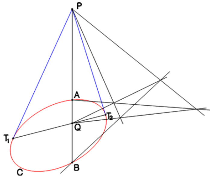
Figura 4. Representación del teorema enunciado donde se demuestra, con la construcción auxiliar de la derecha, que los puntos (P) de concurrencia de las tangentes a la cónica (C) en (T1) y (T2) y (Q), de intersección de la secante transversal (PB) con la cuerda de las tangencias (T1) y (T2), son conjugados armónicos de los puntos (A) y (B) de la cónica (C). La razón doble [P, A, Q, B] = -1
