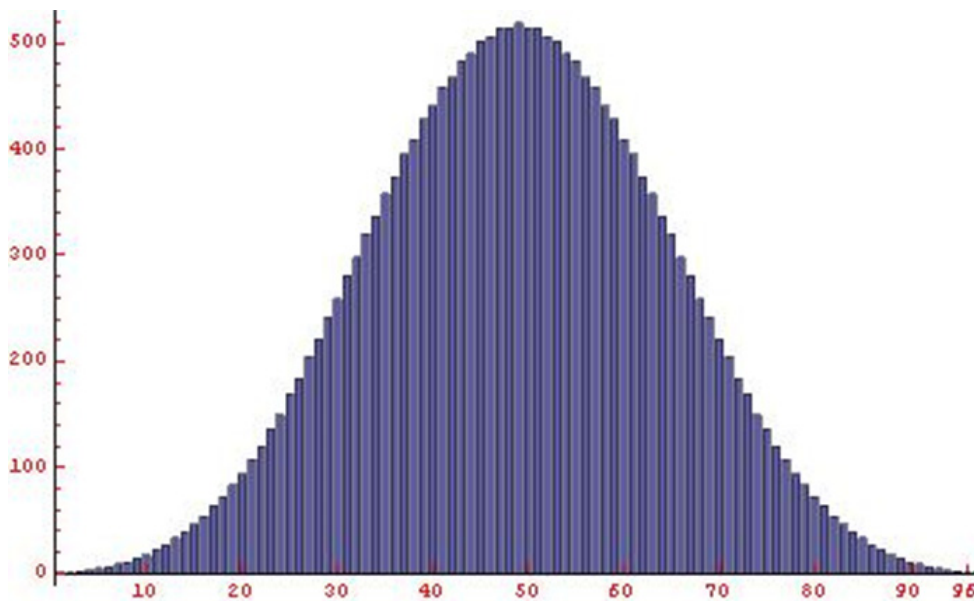
Figura 2. Distribución de la variable aleatoria X_F
