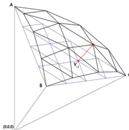
Figura 7. Proyecciones de los vértices del triángulo sobre la esfera.
