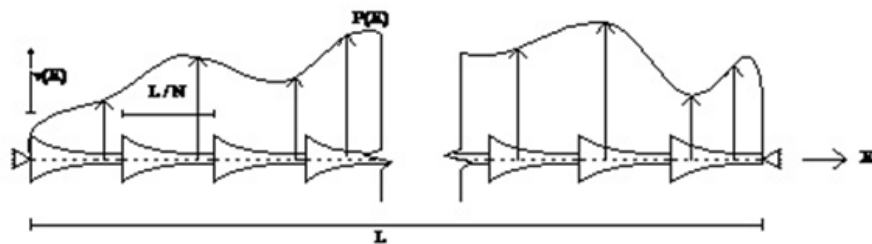
Figura 1. Viga de Bernoulli sometida a una fuerza distribuida vertical y detalle del equilibrio de fuerzas en una rebanada de la misma.
