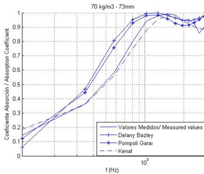
Figura 4 coeficiente de absorción en incidencia normal, comparación entre valores medidos y predichos por distintos modelos. Kenaf 70 kg/m 3 y 73 mm de espesor.
