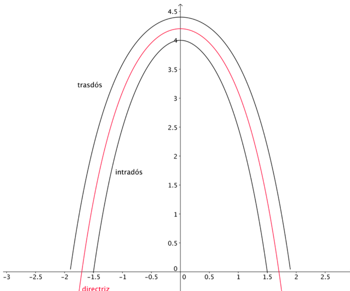
Figura 5: Las curvas del intradós y el trasdós del arco, que no son curvas catenarias, junto con la directriz, que sí lo es. Obsérvese que el intradós cumple las especificaciones de luz, 3 metros, y altura, 4 metros, requeridas.
