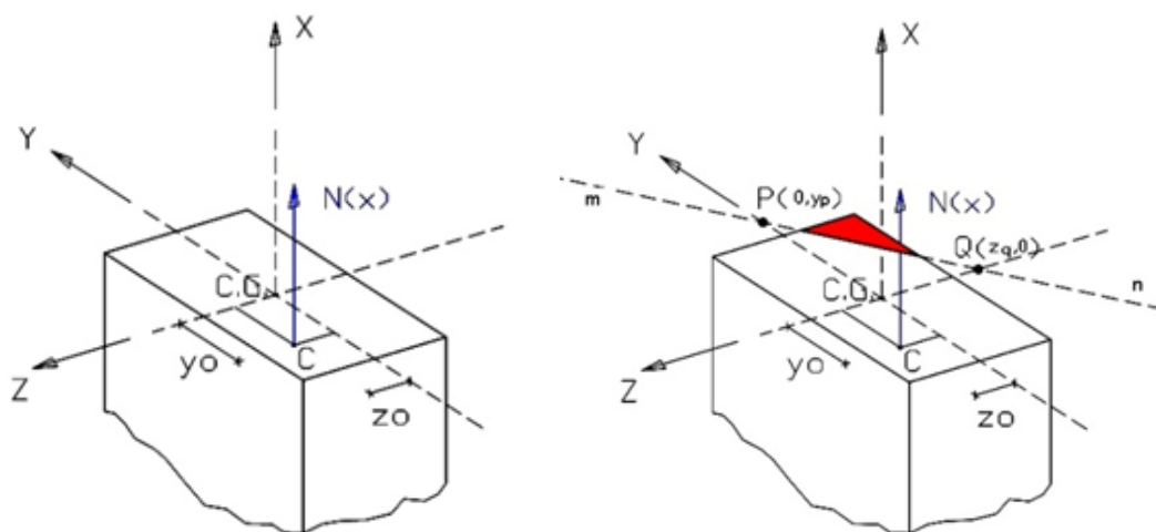
Figura 6. Ubicación del eje neutro ( m-n ) en una sección rectangular, solicitada por una carga axial, N(x) , excéntrica, que origina en ella flexión compuesta.
