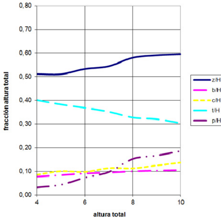
Figura 12 Ábaco de dimensiones normalizadas para un muro
