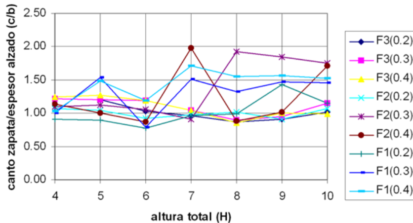
Figura 10 Relación entre la altura total del muro ( H ) y la razón entre el canto de la zapata y el espesor del alzado ( c/b ), en función del tipo de relleno
