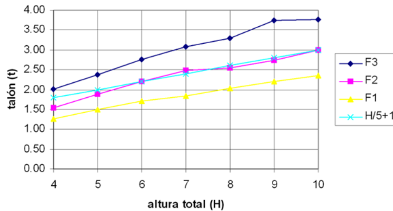
Figura 9 Relación entre la altura total del muro ( H ) y la longitud del talón ( t ), en función de la capacidad portante del suelo y del criterio de predimensionamiento t \approx H/5 + 1
