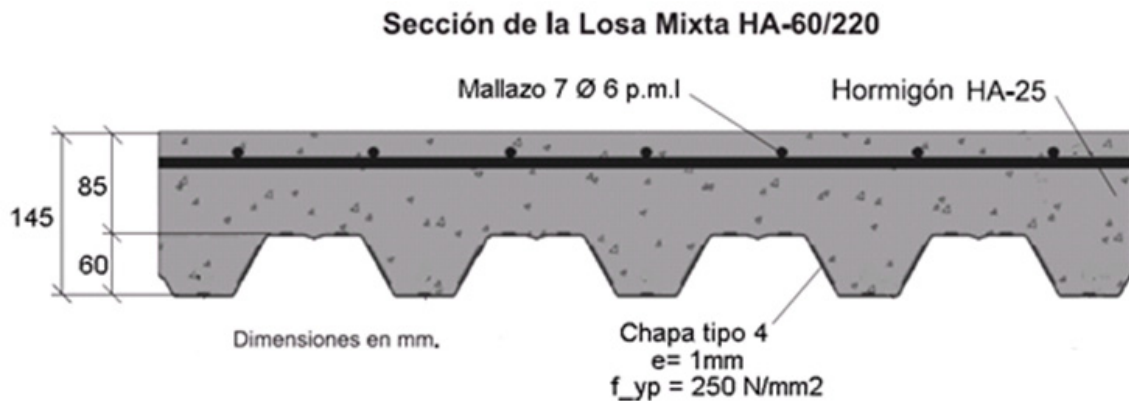
Figura 6 Forjado óptimo para una luz de 3,50m.
