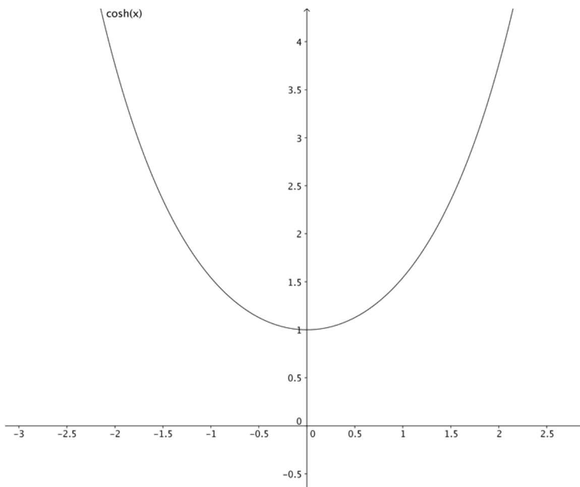
Figura 2: Gráfica de la función coseno hiperbólico.
