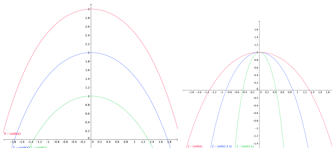
Figura 3: Variedad de gráficas de la función coseno hiperbólico. En la izquierda se varía el término constante. En la derecha se varía la escala de medida de x.
