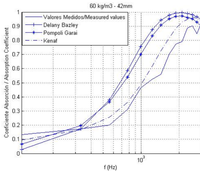
Figura 5 coeficiente de absorción en incidencia normal, comparación entre valores medidos y predichos por distintos modelos. Kenaf 60 kg/m 3 y 42 mm de espesor.
