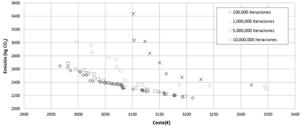
Figura 2. Coste frente emisión de CO 2 . Evolución de la frontera de Pareto
