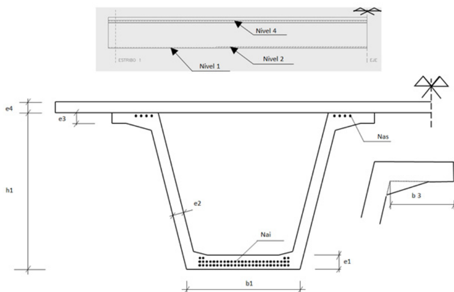
Figura 3. Variables y parámetros geométricos. Alzado y sección
