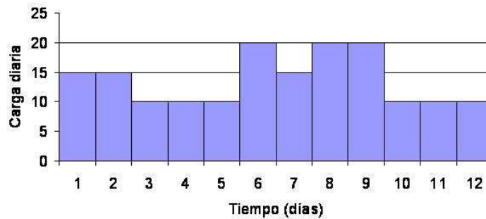
Figure 10: Calendario de ejecución y diagrama de cargas (nivelación final)
