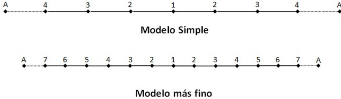
Figura 4. Distribución de los nodos para carga puntual en viga Bernoulli biapoyada.
