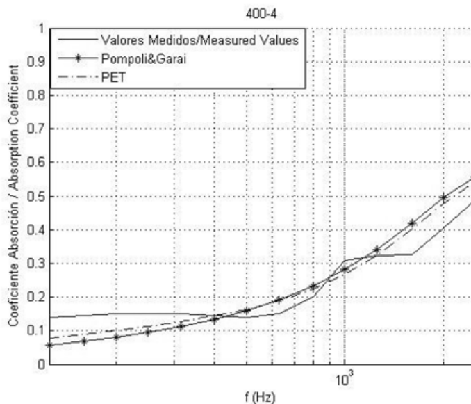
Figura 6 coeficiente de absorción en incidencia normal, comparación entre valores medidos y predichos por distintos modelos. Poliéster Reciclado 1200 g/m 2 y 40 mm de espesor
