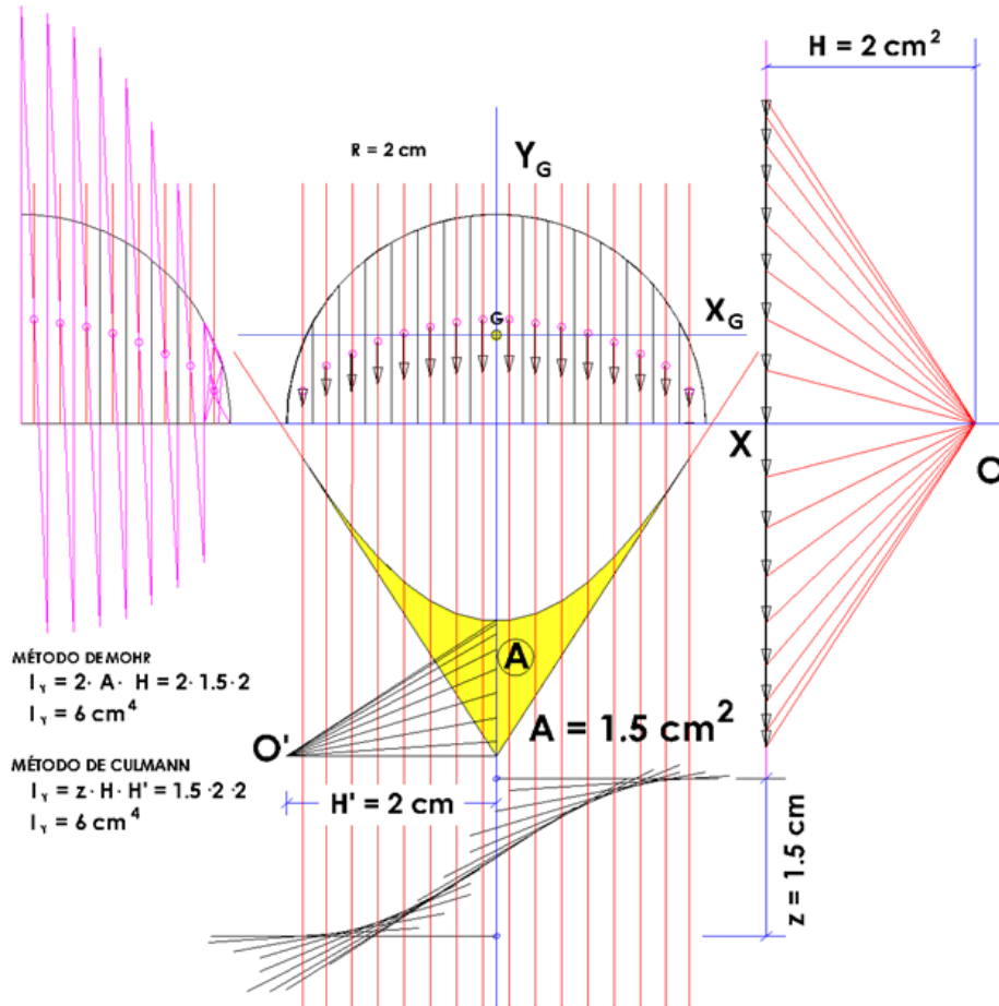
Figura 10. Cálculo del Momento de Inercia de un semicírculo de radio 2 cm respecto a su Eje de Simetría, mediante el método Culmann y el método de Mohr del Área encerrada entre el funicular y el Eje de Momentos.
