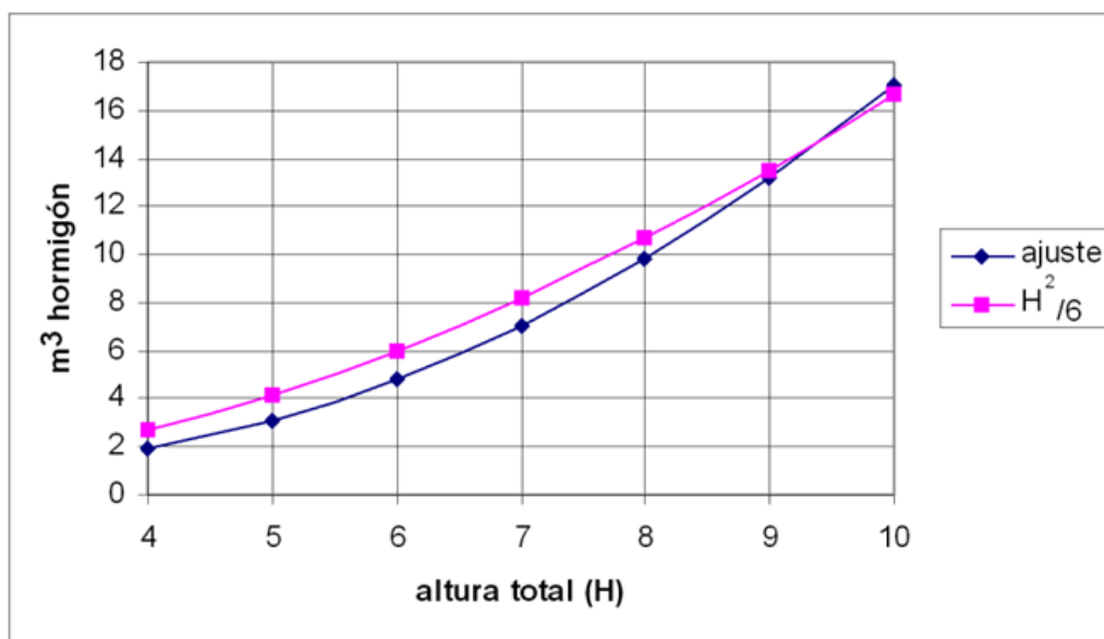
Figura 4 Relación entre la altura total del muro (H) y el volumen de hormigón, tanto con el ajuste como por el predimensionamiento propuesto
