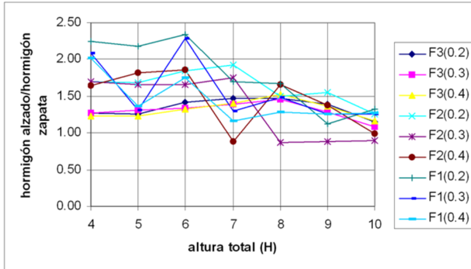
Figura 5 Relación entre la altura total del muro (H) y el ratio del volumen de hormigón necesario en alzado y en zapata
