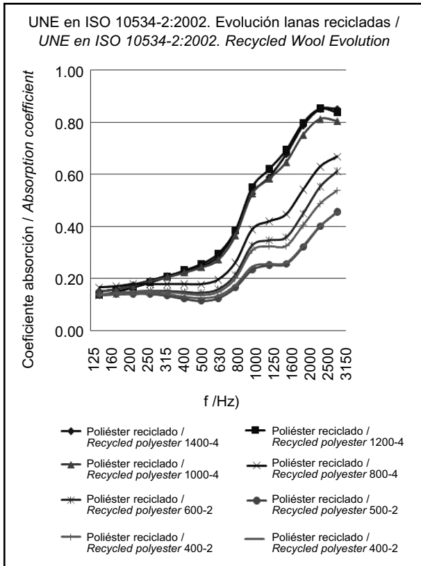
Figura 3. Coeficiente de absorción en incidencia normal para muestras de Poliéster reciclado. Figure 3. Absorption coefficient in normal incidence for samples of recycled polyester.
