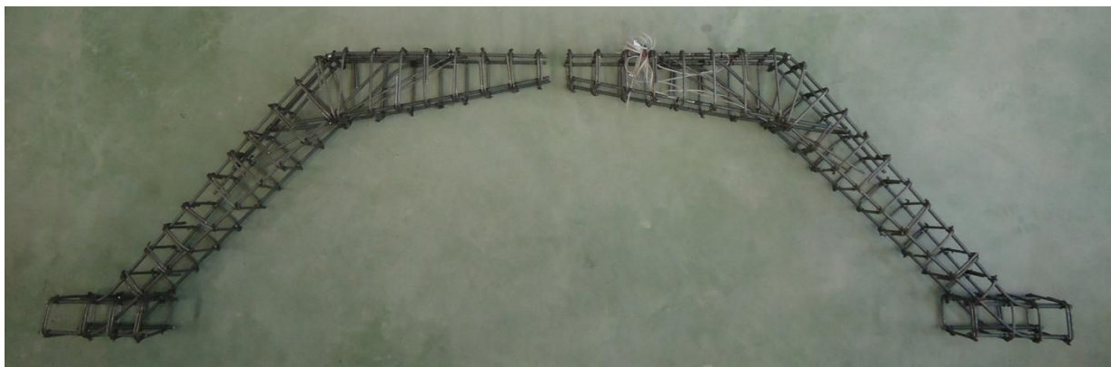
Figura 8.13. Ferralla armada del elemento diseñado.
