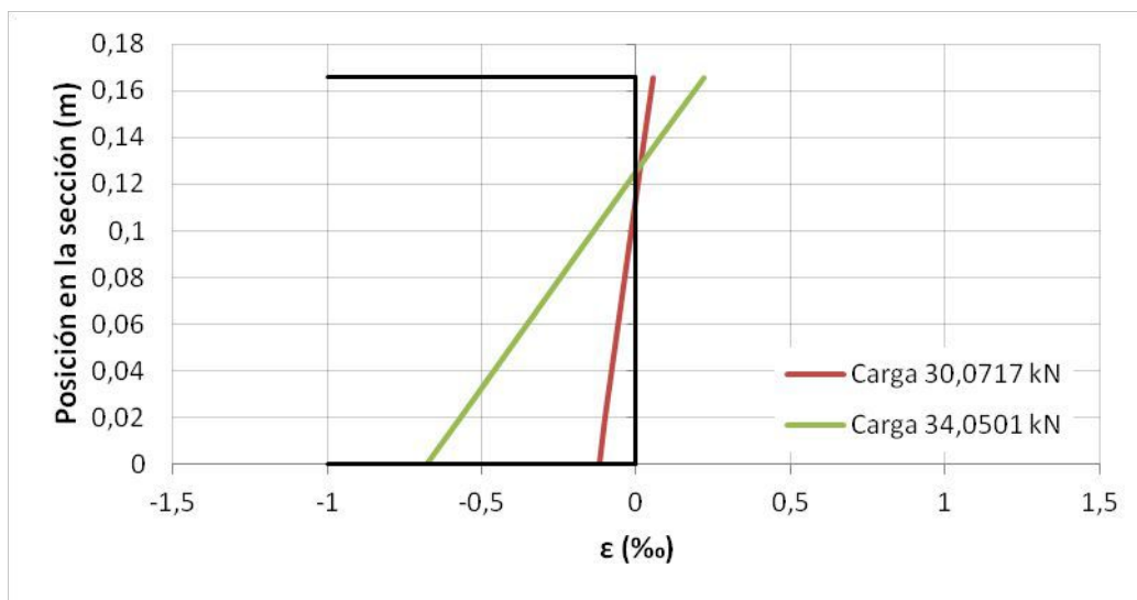
Figura 10.50. Representación del plano de deformaciones de la sección G en el ensayo 1 mediante los datos de deformaciones obtenidos del ensayo.
