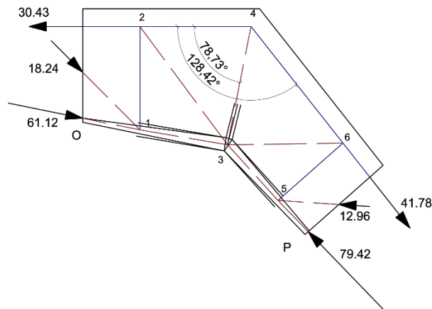
Figura 4.26. Tercer modelo de bielas y tirantes propuesto para la región OP en el cual se modifican los brazos mecánicos en las secciones O y P y se desplaza el nudo 3. Representación de los anchos de las bielas y el nudo que forman.
