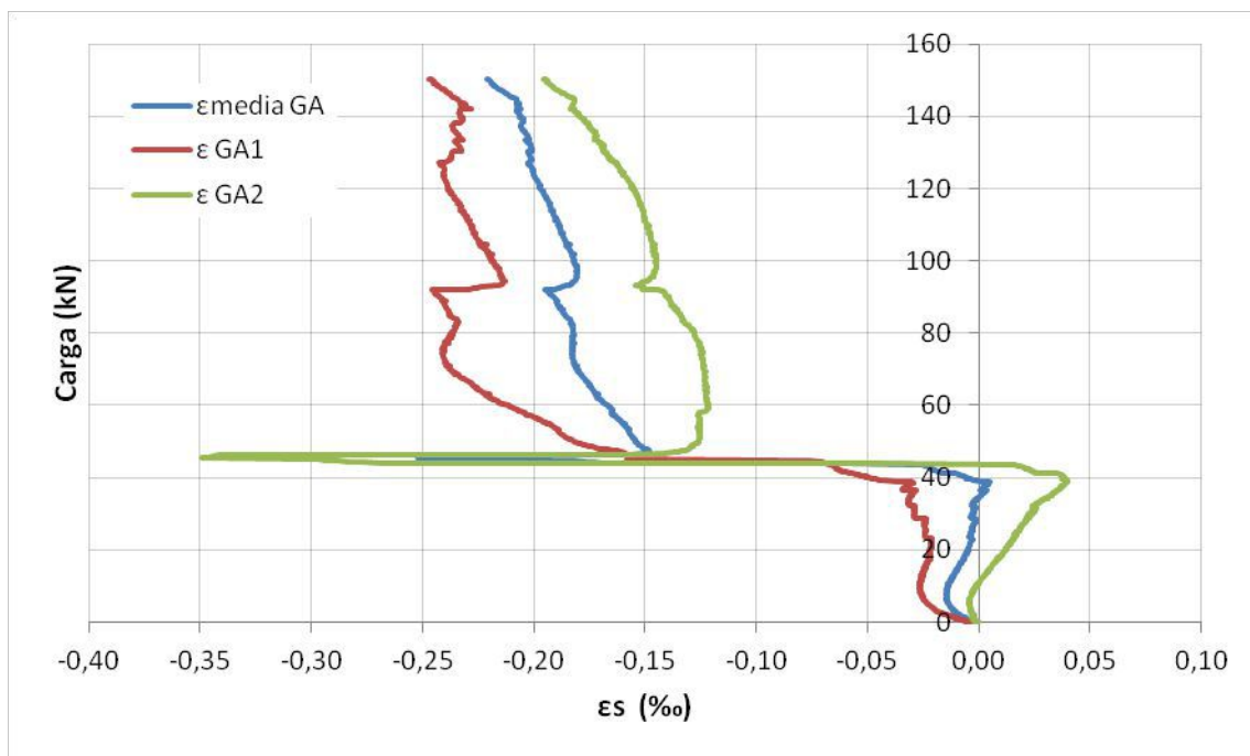
Figura 10.40. Gráfica carga-deformación medida por las galgas GA en el ensayo 2.
