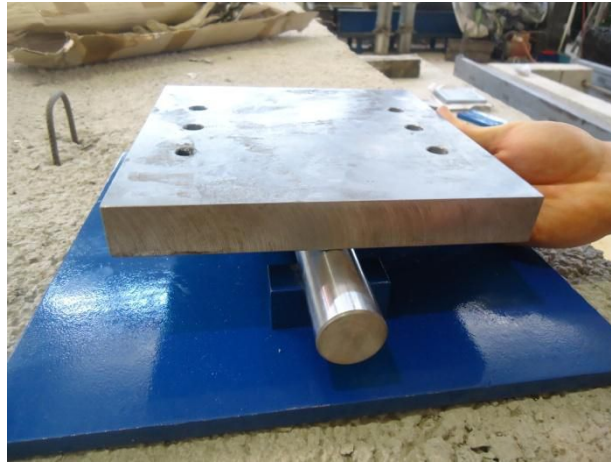
Figura 6.3. Aparato de apoyo.
