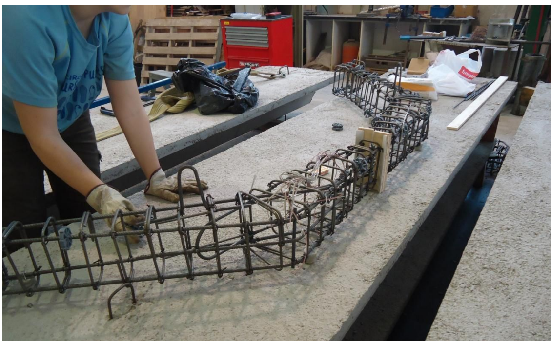
Figura 8.18. Colocación de los separadores en la pieza y fijación del encofrado de la rótula.
