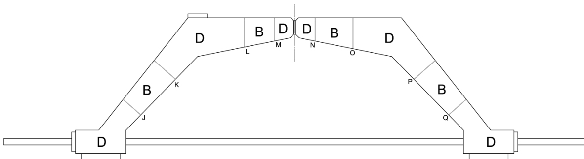
Figura 4.8. Regiones B y D del elemento.
