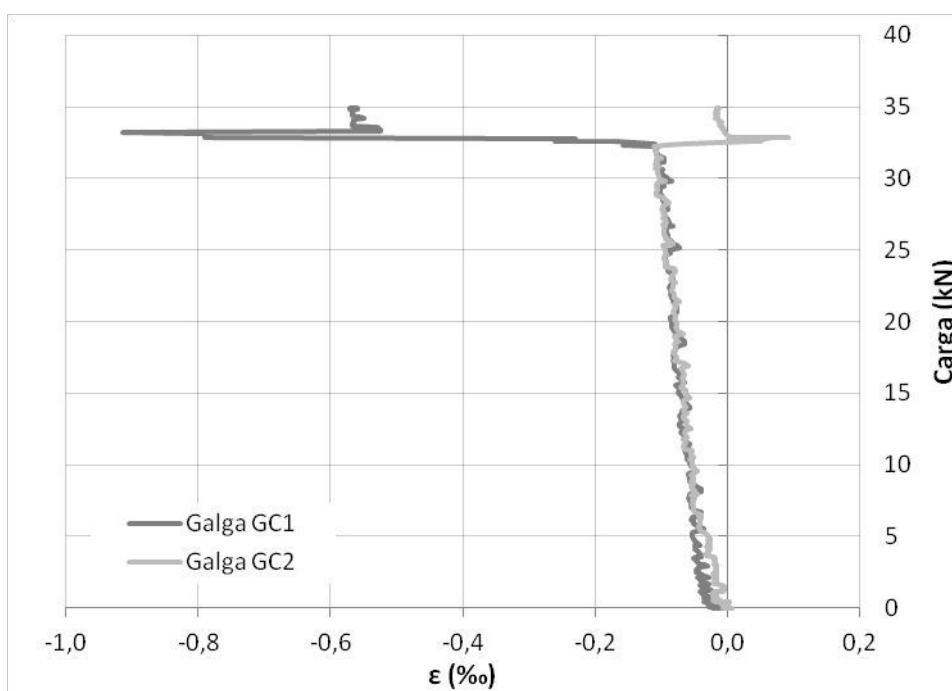
Figura 10.44. Gráfica carga-deformación medida por las galgas GC en el ensayo 1.
