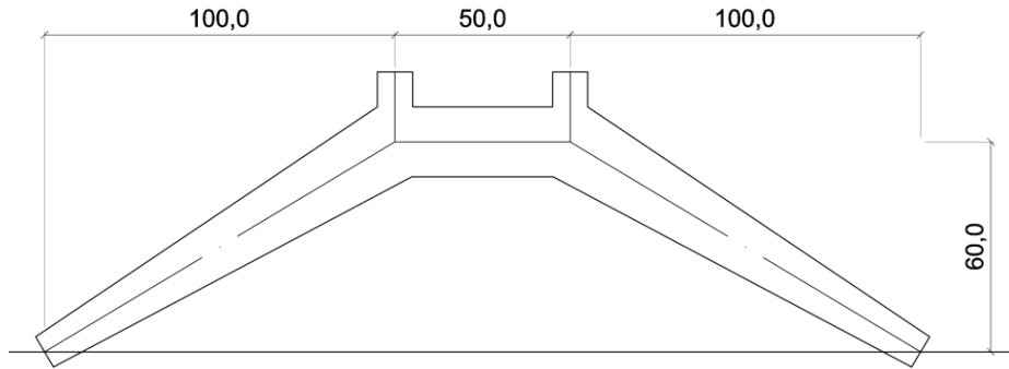
Figura 3.2. Geometría inicialmente propuesta.
