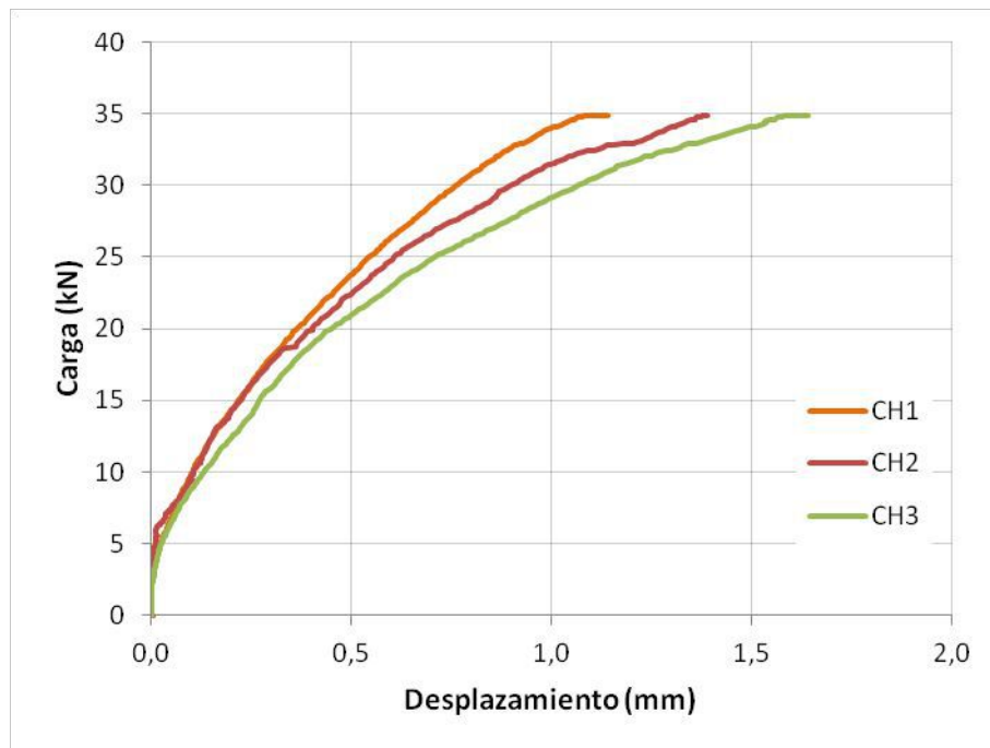
Figura 10.23. Gráfica carga-desplazamiento horizontal medido por los captadores en el ensayo 1.
