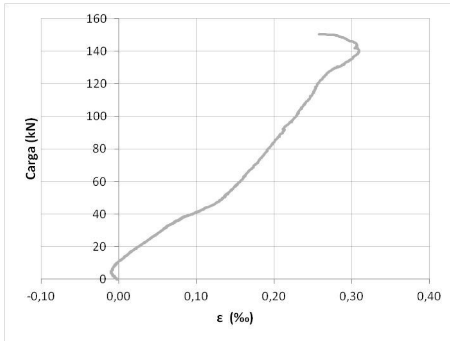
Figura 10.55. Gráfica carga-deformación medida por la galga GB1 en el ensayo 2.
