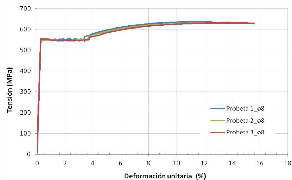
Figura 5.24. Gráfica tensión-deformación unitaria de las barras ø8 ensayadas.
