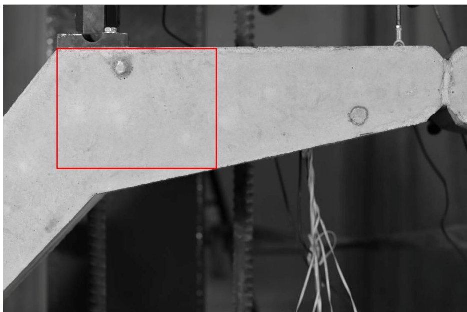
Figura 10.24. Región situada bajo la rótula de carga estudiada mediante fotogrametría.
