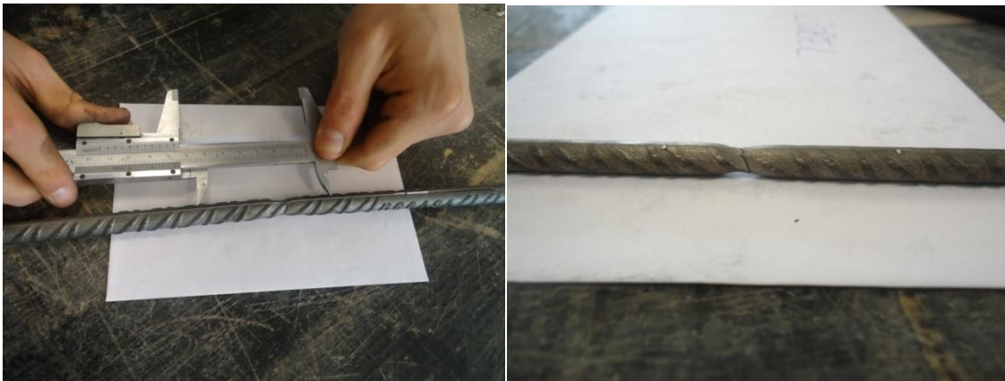
Figura 5.21. a) Medición de la probeta tras el ensayo para el cálculo del alargamiento en rotura; b) Estricción sufrida por la barra en la zona de rotura.
