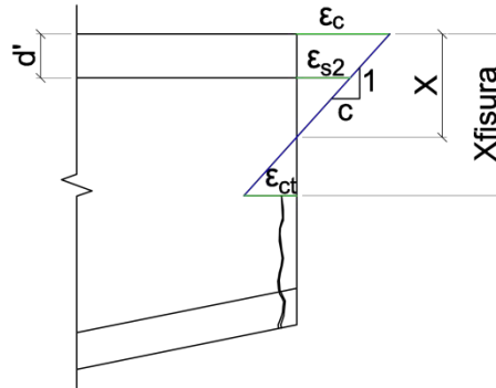
Figura 10.49. Esquema del plano de deformaciones de la sección tras la fisuración.
