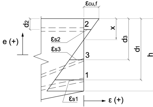
Figura 11.3. Plano de deformaciones considerado en el modelo de rotura.
