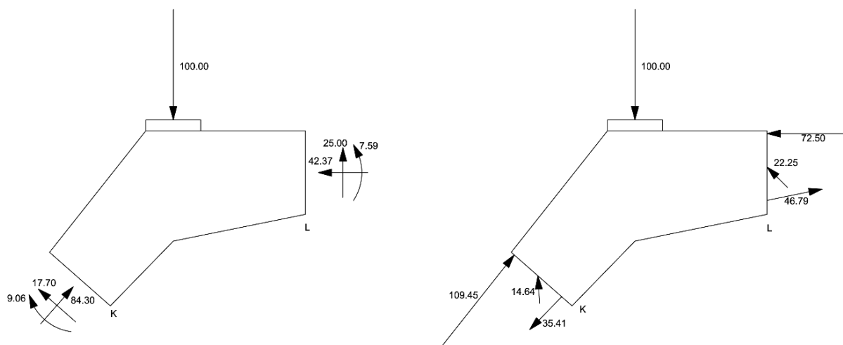
Figura 4.11. a) Esfuerzos en la región KL; b) Sistema equivalente de fuerzas puntuales en la región KL.
