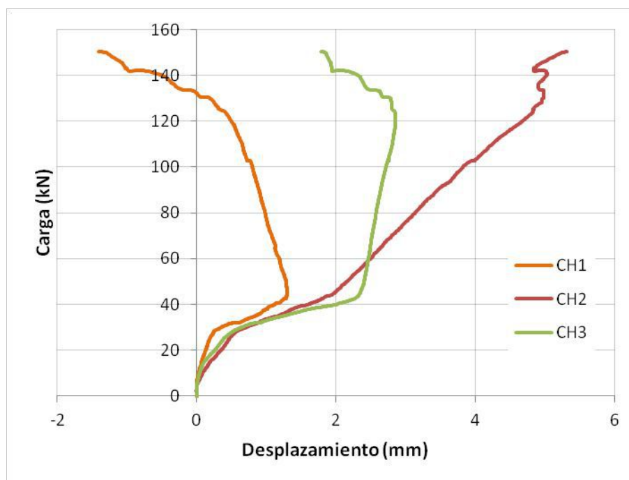
Figura 10.22. Gráfica carga-desplazamiento horizontal medido por los captadores en el ensayo 2.
