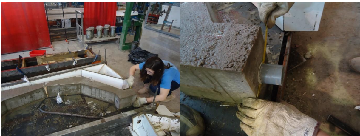
Figura 8.27. a) Desencofrado de la estructura; b) Corte del tramo sobrante de los tubos de PVC.
