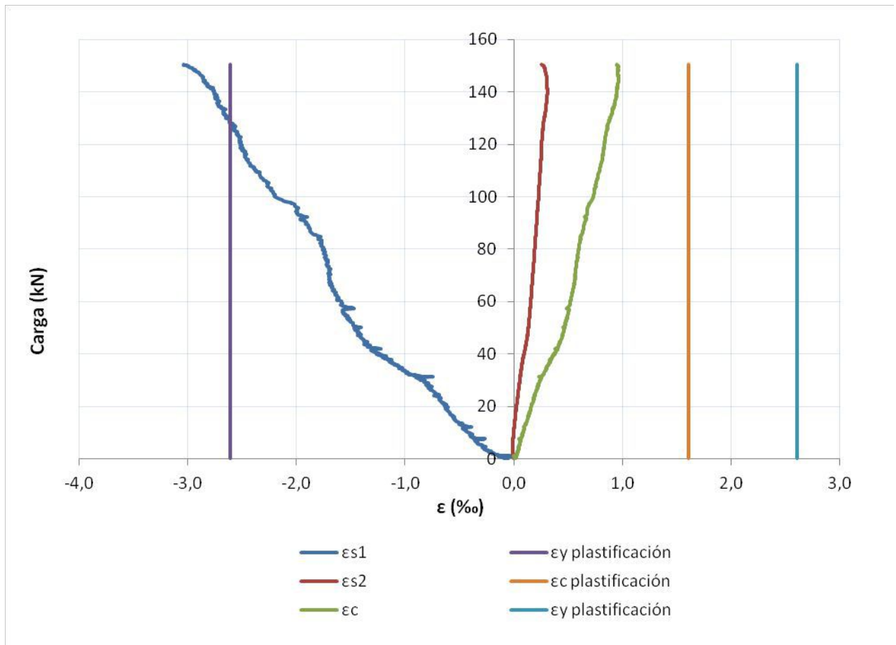
Figura 10.45. Gráfica carga-deformaciones en la sección G en el ensayo 2.
