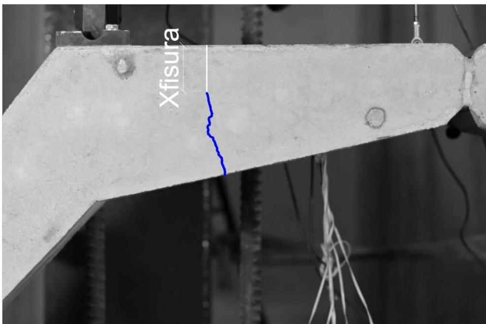
Figura 10.48. Medida de la profundidad de la fisura mediante fotogrametría (sección G).
