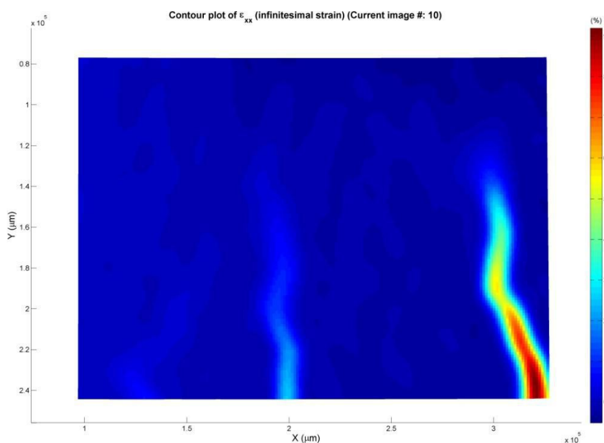
Figura 10.36. Deformaciones unitarias del hormigón en la dirección x para 147 kN de carga en el ensayo 2.
