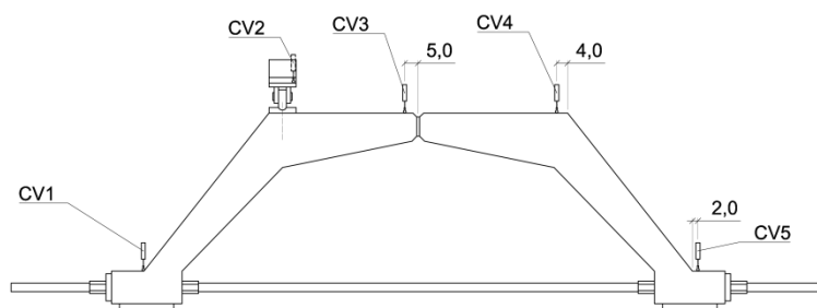
Figura 10.27. Posición de los captadores de desplazamiento vertical.
