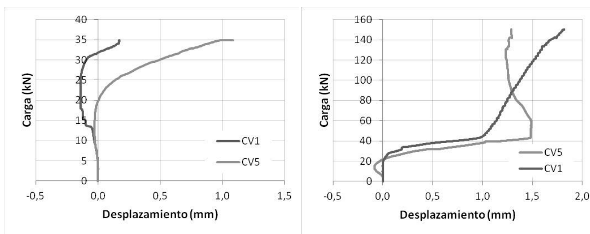
Figura 10.28. a) Gráfica carga-desplazamiento vertical medido por los captadores de los apoyos en el ensayo 1; b) Gráfica carga-desplazamiento vertical medido por los captadores de los apoyos en el ensayo 2.
