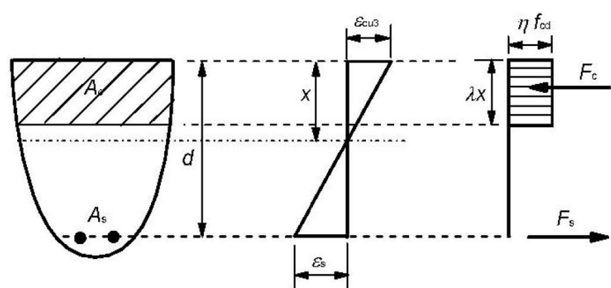
Figura 4.5. Diagrama rectangular de la tensión en el hormigón. [9]
