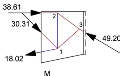
Figura A.9. Modelo de bielas y tirantes propuesto para la región M.
