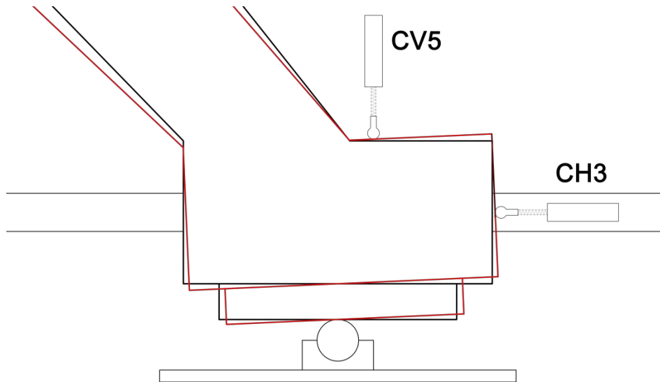
Figura 10.20. Representación del giro que sufre el apoyo según las medidas de los captadores.
