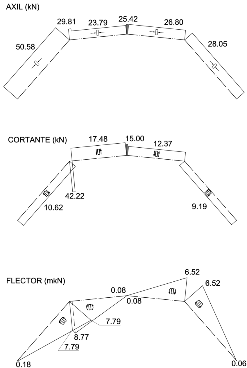
Figura 4.29. Leyes de esfuerzos para la verificación de los ELS.
