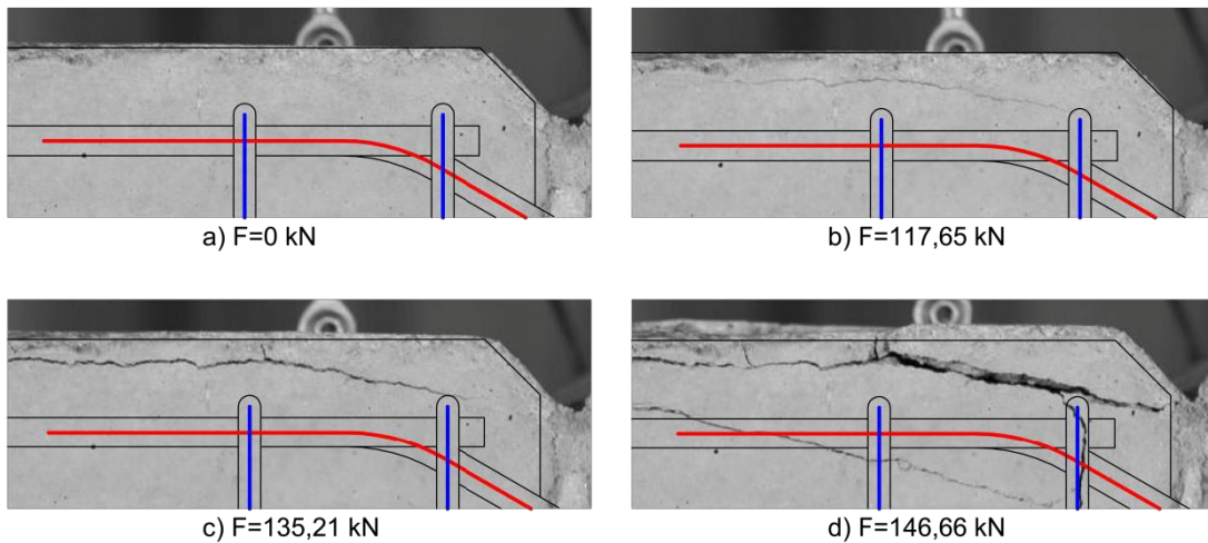
Figura 11.18. Fotografías del proceso de rotura de la región sobre las que se monta el armado dispuesto.
