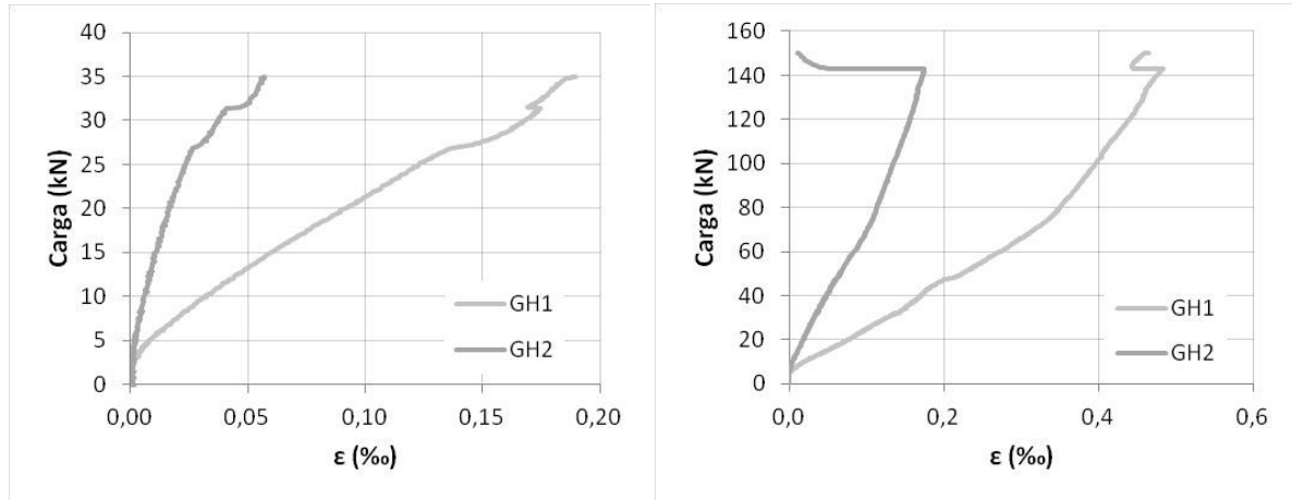
Figura 10.38. a) Gráfica carga-deformación medida por las galgas GH1 y GH2 en el ensayo 1; b) Gráfica carga-deformación medida por las galgas GH1 y GH2 en el ensayo 2.
