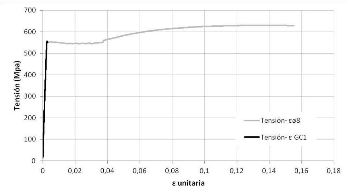
Figura 10.47. Superposición de la gráfica tensión-deformación medida por la galga GC1 en el ensayo 2 y la ecuación constitutiva de un Ø8.
