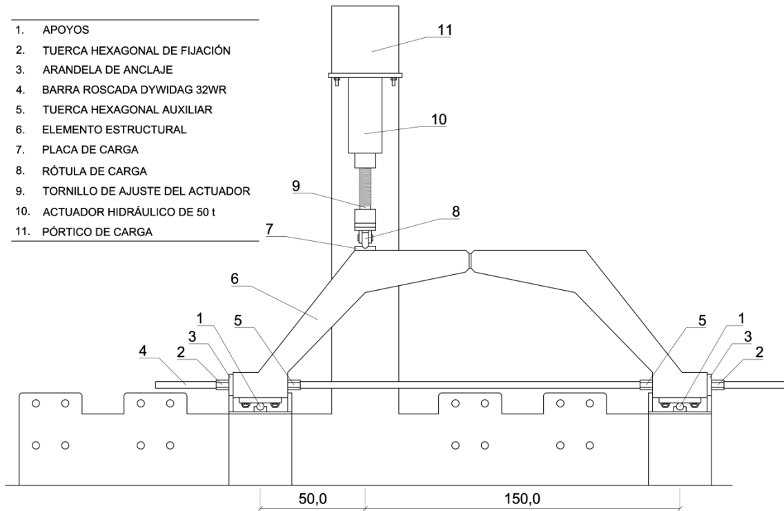
Figura 6.1. Montaje para el ensayo sin instrumentación.
