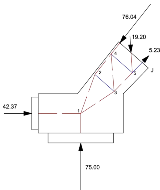
Figura A.5. Modelo de bielas y tirantes propuesto para la región J.
