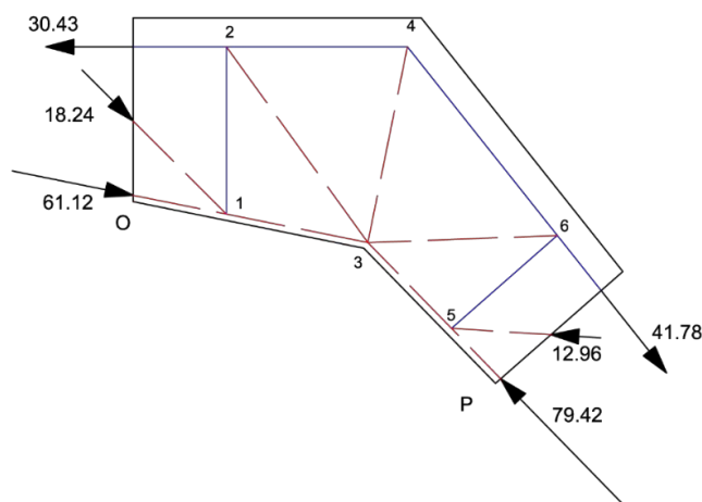
Figura 4.23. Segundo modelo de bielas y tirantes propuesto para la región OP en el cual se modifican los brazos mecánicos en las secciones O y P.
