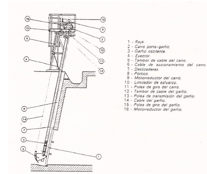
Ilustración 1. Rejilla con dispositivo automático de limpieza
