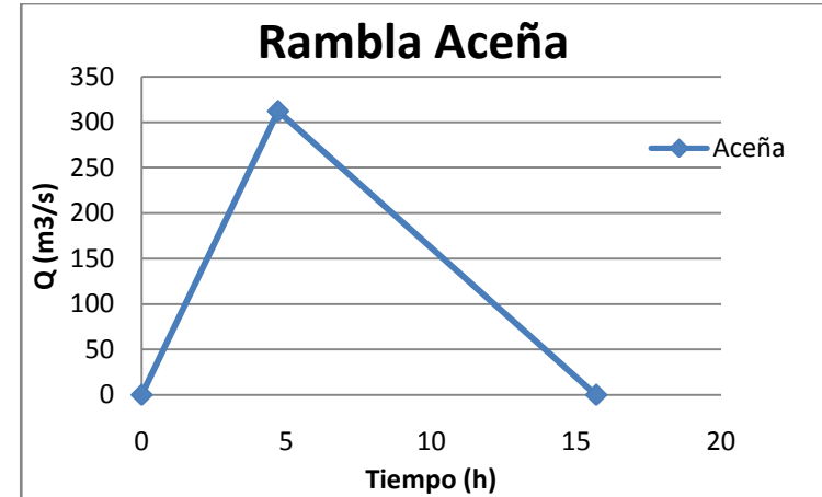
Ilustración 10. Hidrograma unitario Rambla Aceña. Captación 1
