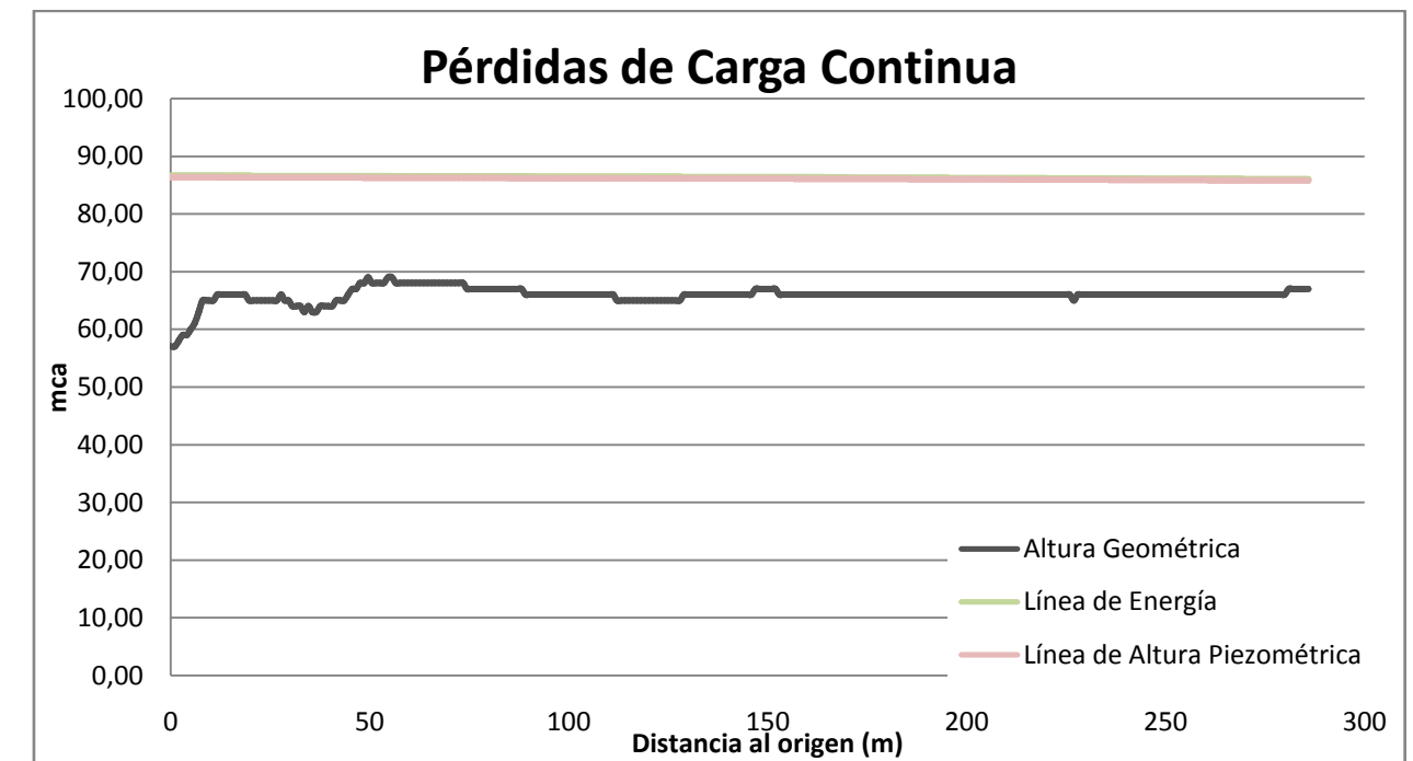
Figura 3: Gráfico Pérdidas Continuas, Cámara de Reparto 3.
