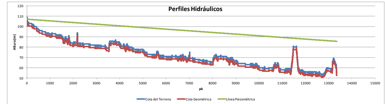
Ilustración 9. Línea de alturas piezométricas. Tubería. C1.
