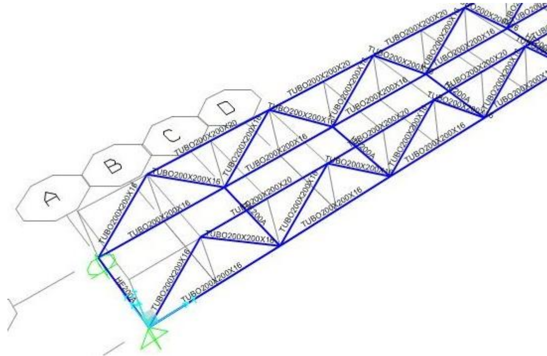
Ilustración 3: Cercha
