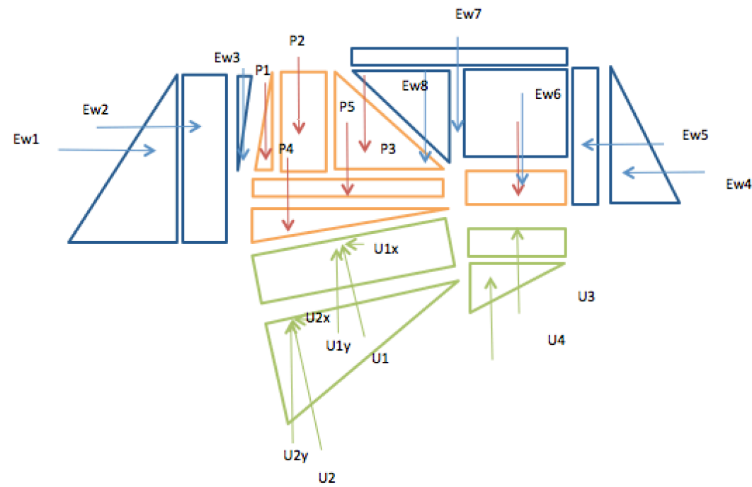
Ilustración 3. Fuerzas resultantes
