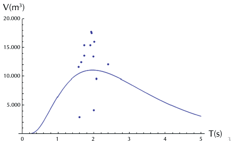
3. Volumen óptimo según el modelo estudiado, para distintos tiempos de reverberación. Los puntos corresponden a las salas estudiadas en (6).
