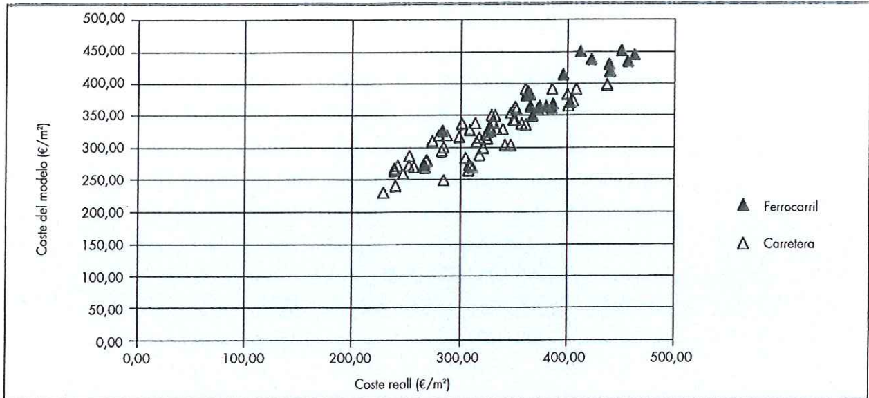
FIGURA 8. Relación entre el coste real y el estimado por el modelo para las losas de ferrocarril y de carreteras.
