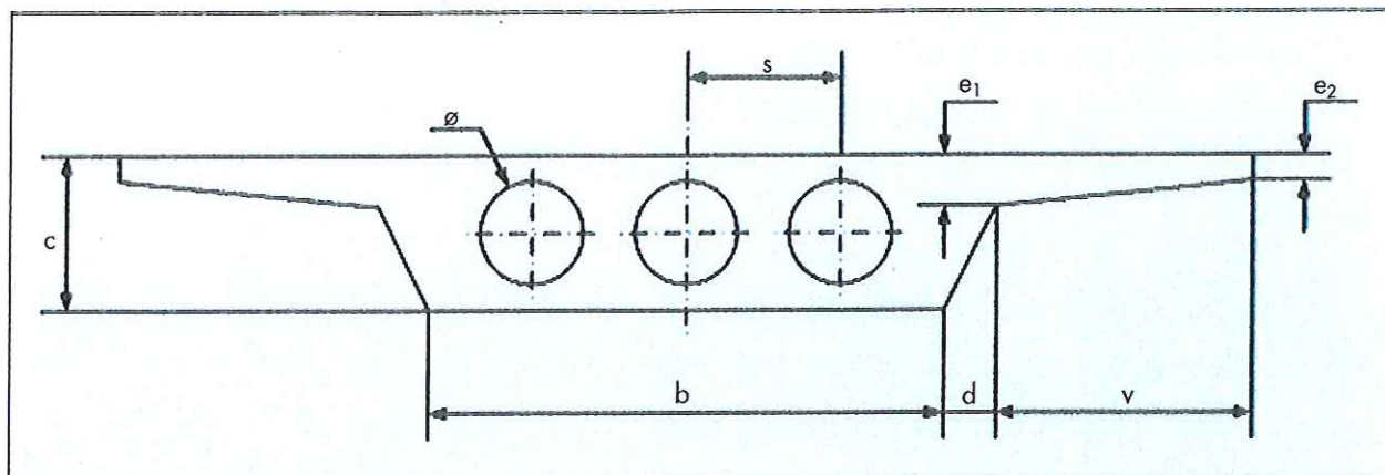
FIGURA 1. Sección tipo de tablero de puente losa en "ala de gaviota" y aligeramientos.
