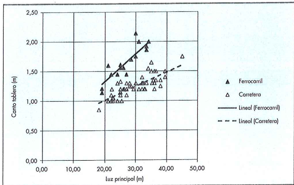
FIGURA 5. Relación entre la luz principal y el canto del tablero.
