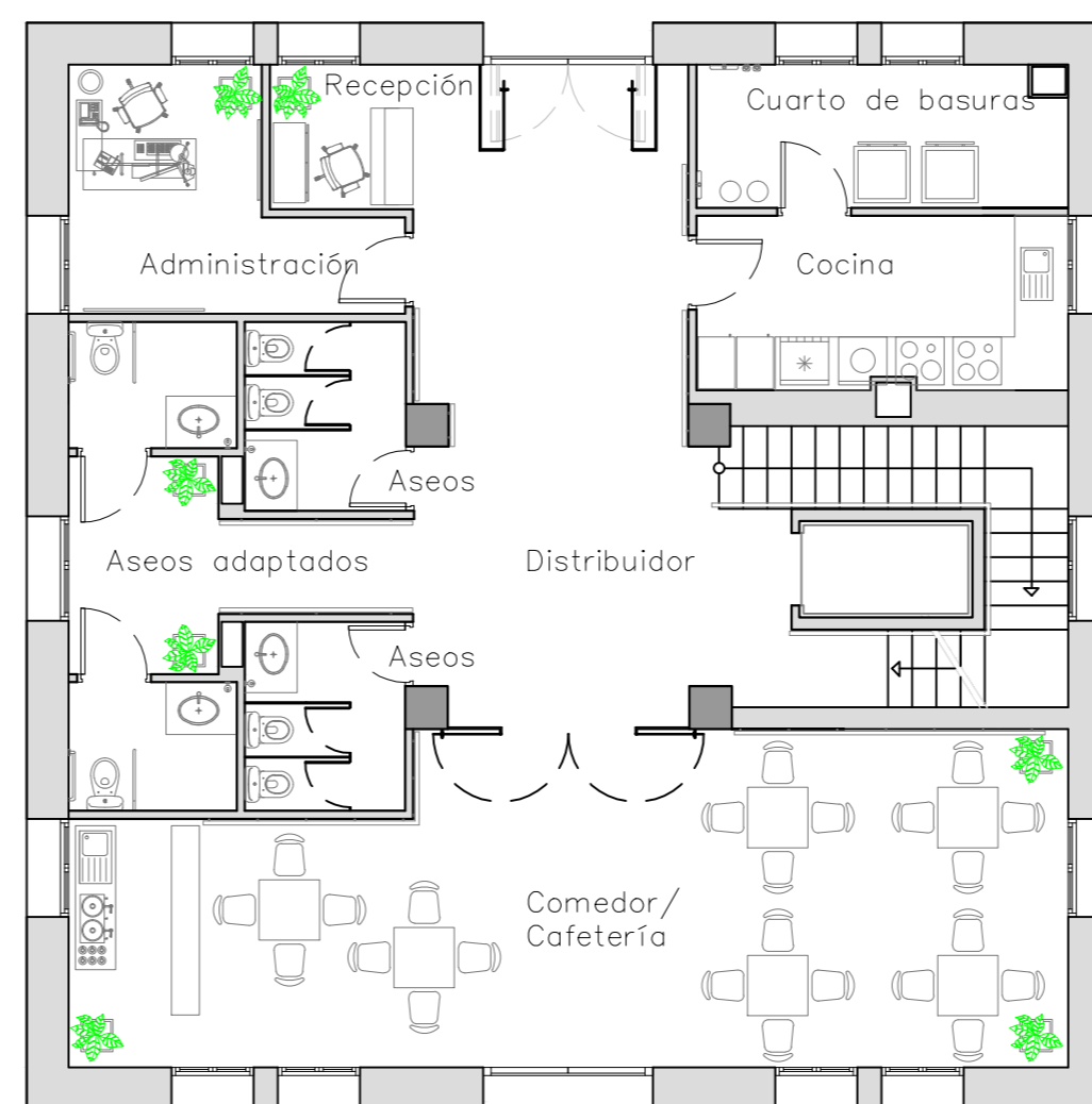
Planta Baja
