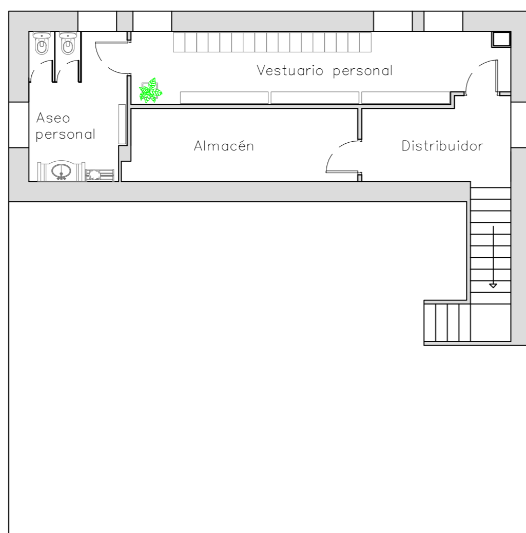
Planta Sótano
