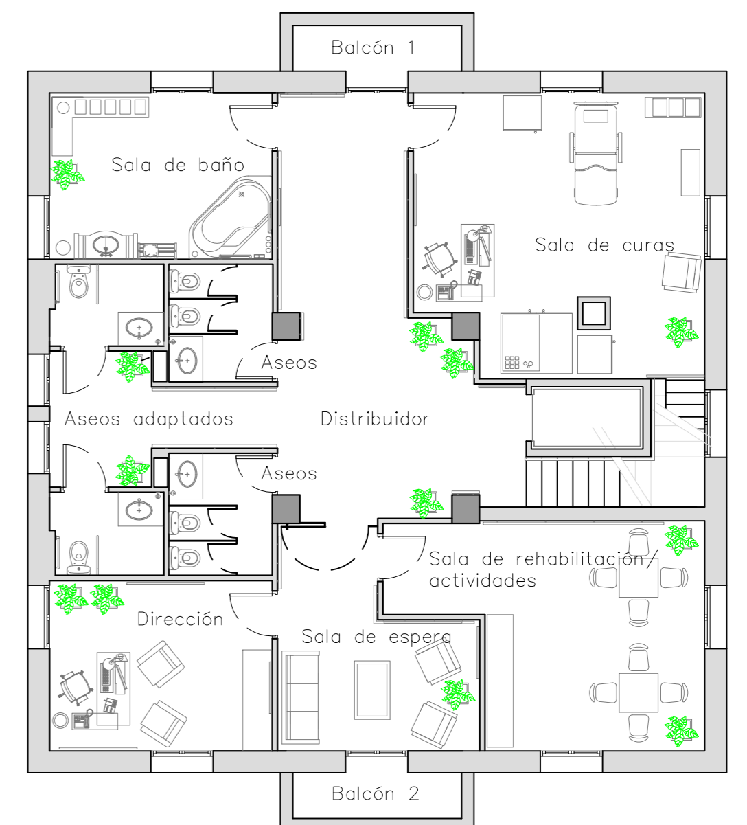
Planta Primera
