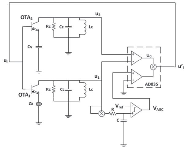
Figura 2 Diagrama del sistema propuesto para la caracterización de la microbalanza de cristal de cuarzo (QCM)
