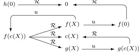
Figura 4.1: Grafo de dependencias entre términos \mathcal{I}_{\mathcal{R}} .
