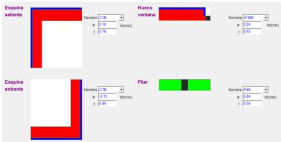
Figura5 y 6 puentes térmicos
