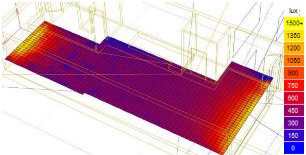
Cálculos Ecotec, inclinación 15º Planta Baja, DL Iluminancia interior.
