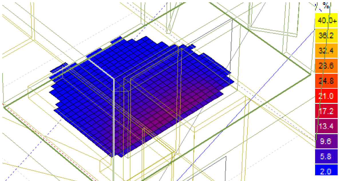
Cálculos Ecotec, inclinación 15º Planta Segunda, DF Factor de iluminación natural (FIN).
