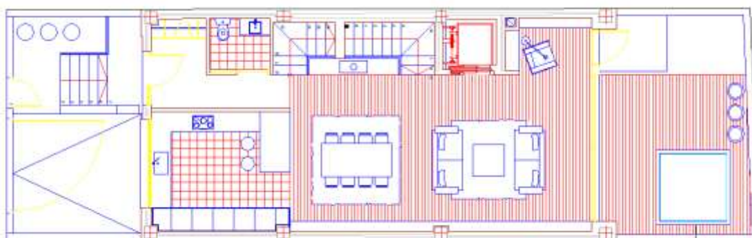
PLANTA BAJA
