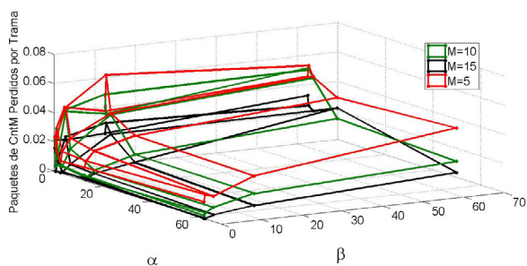
Figura 13: Paquetes de CntM perdidos en promedio por trama en función de \alpha , \beta y M .
