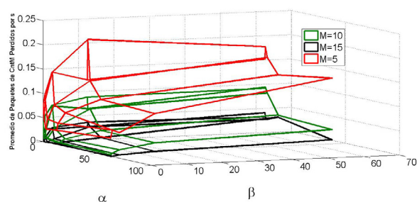
Figura 14: Paquetes de CntM perdidos en promedio por unidad de tiempo en función de \alpha , \beta y M .
