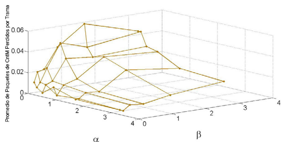
Figura 10: Promedio de paquetes de CntM perdidos por trama, \bar{L}_{CntM} en función de \alpha y \beta .
