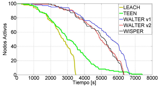
Figura 2: Tiempo de vida de la red
