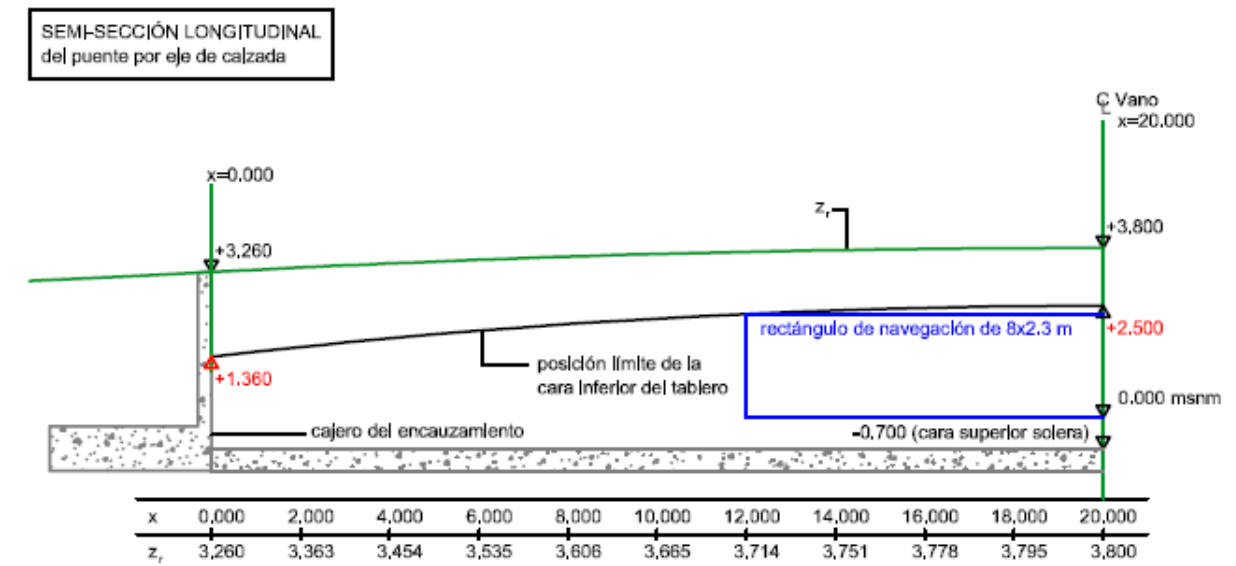
Figura 6 Semi-sección longitudinal de gálibos exigidos
