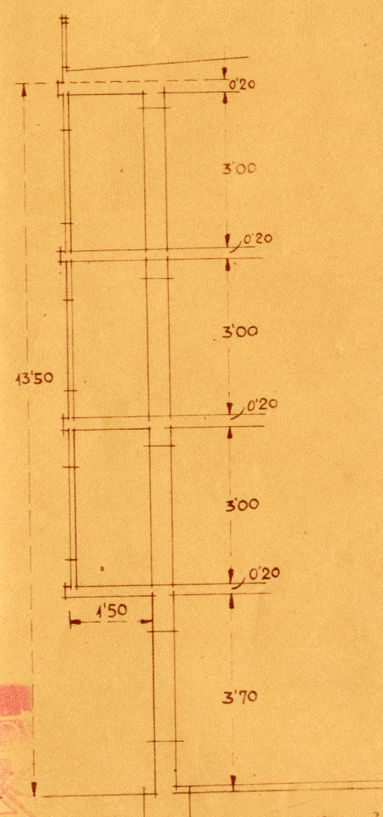
Sección A.B.
