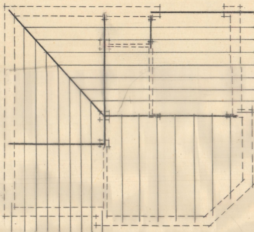
Entramado de cubierta
