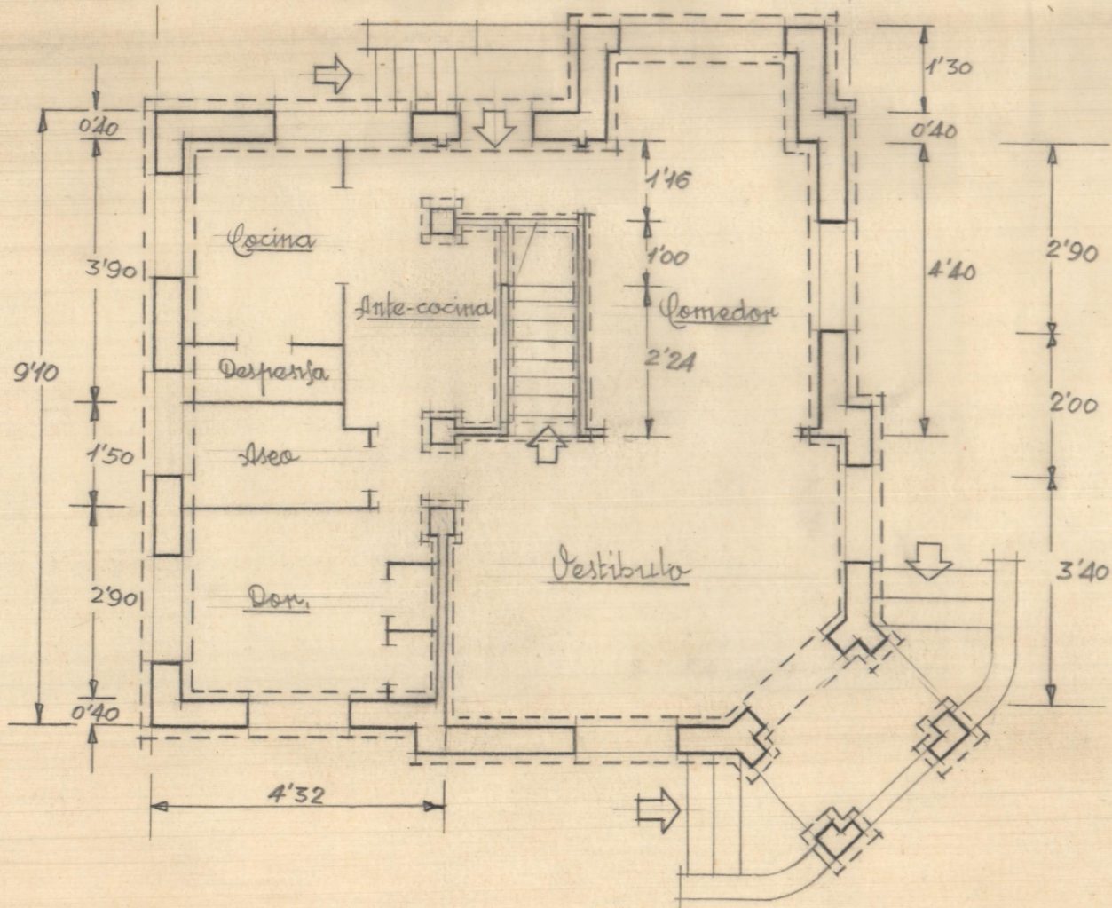
Planta baja y cimientos
