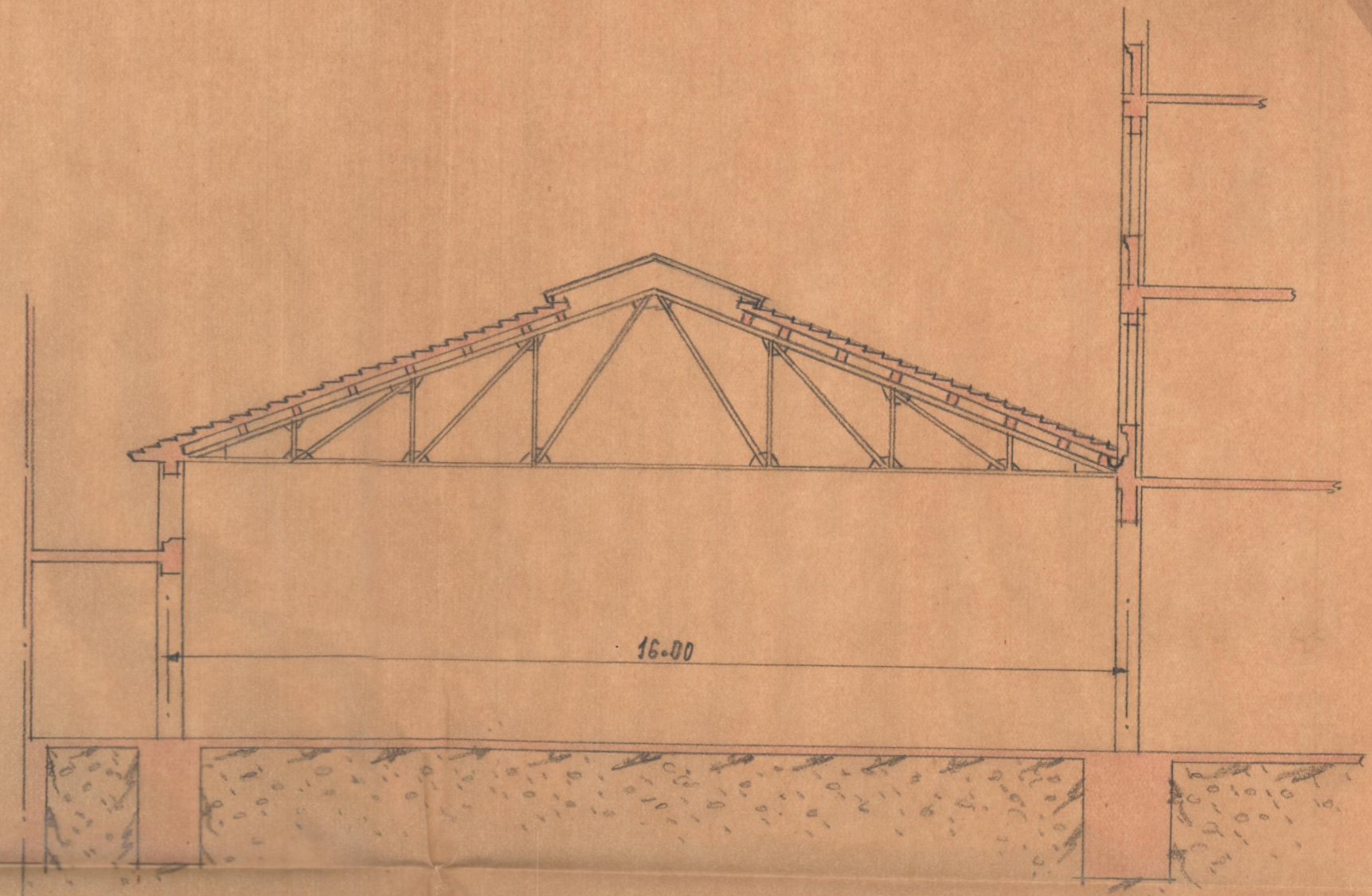
Cubierta interior Sección por C.D.
