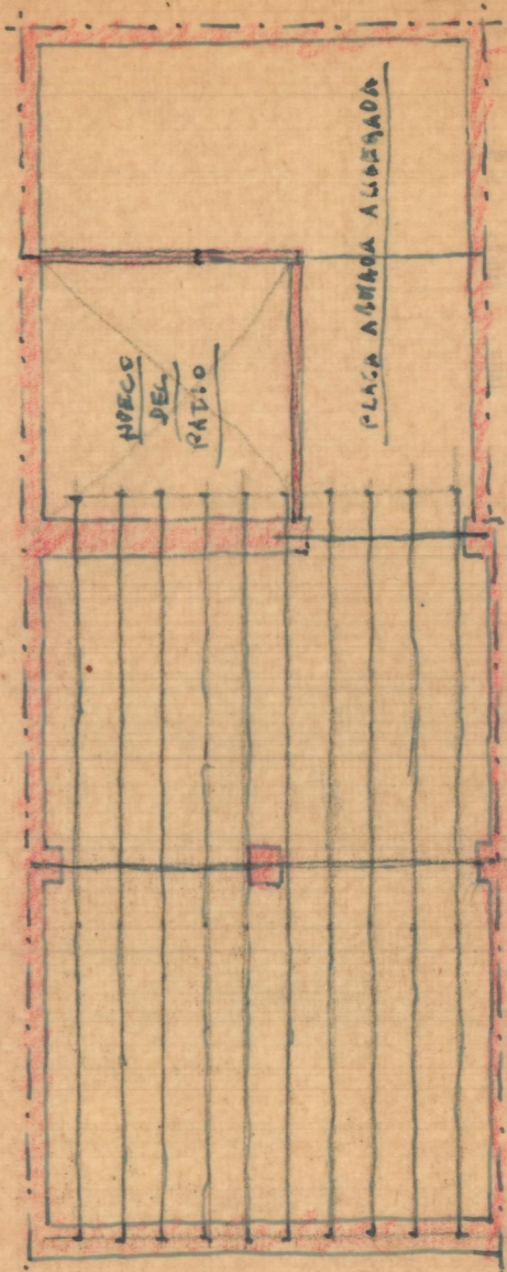
ENTRANADO DE COBIERTA
