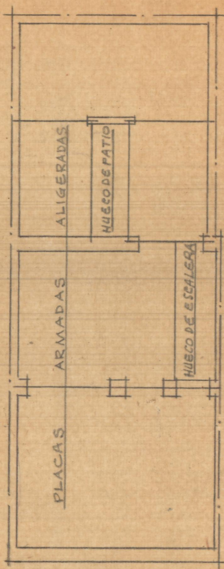
Entramado de piso
