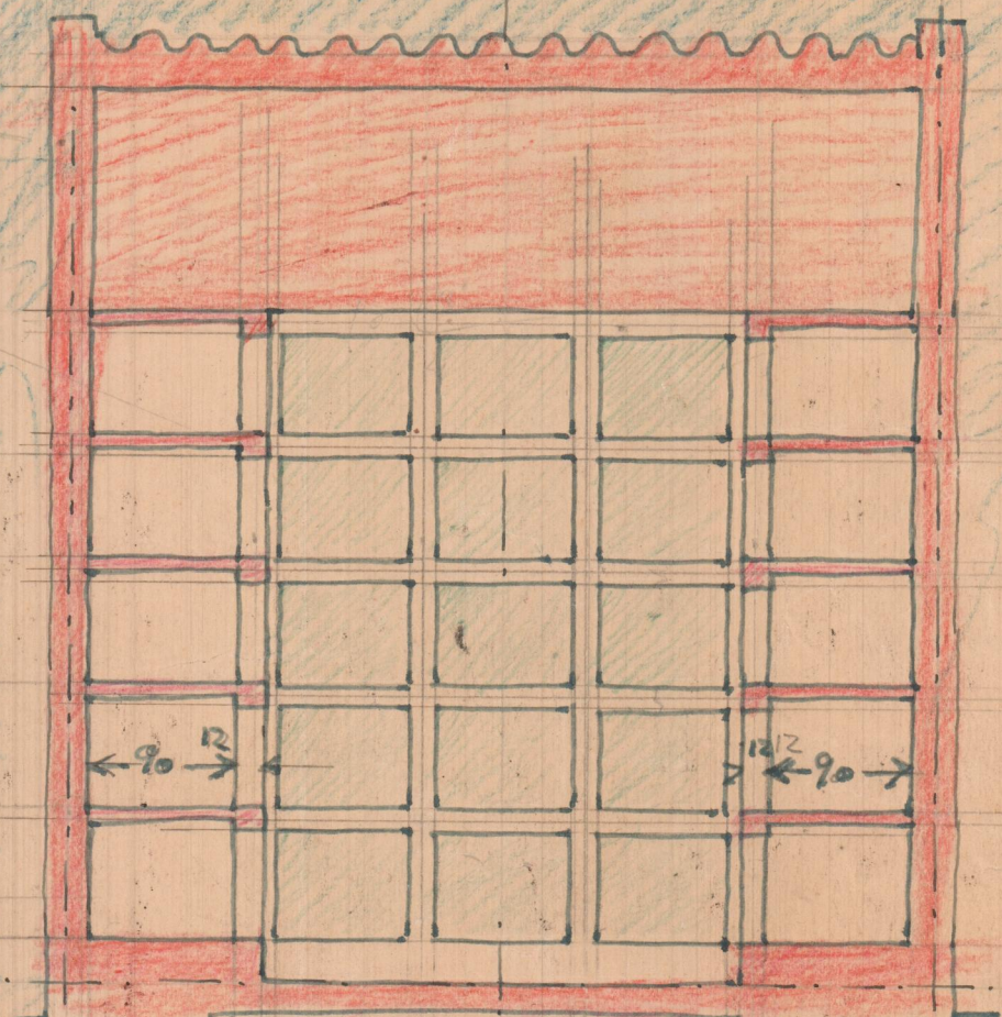
SECCION TRANSVERSAL AB
