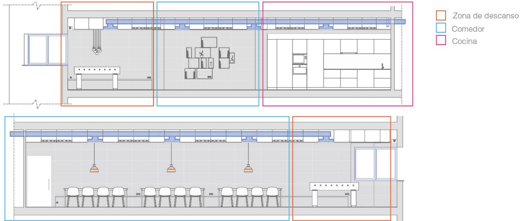
Secciones Cocina
