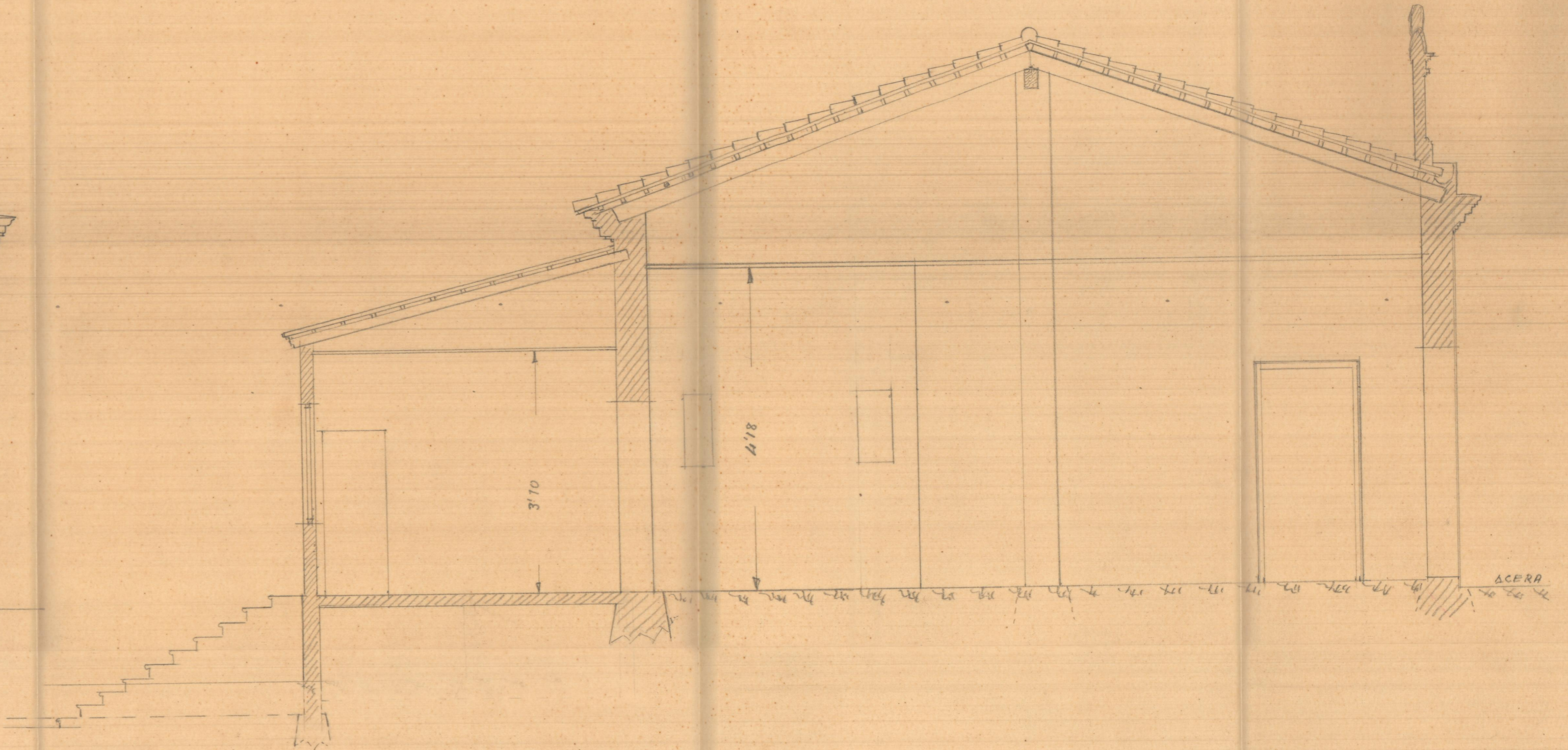
SECCION
