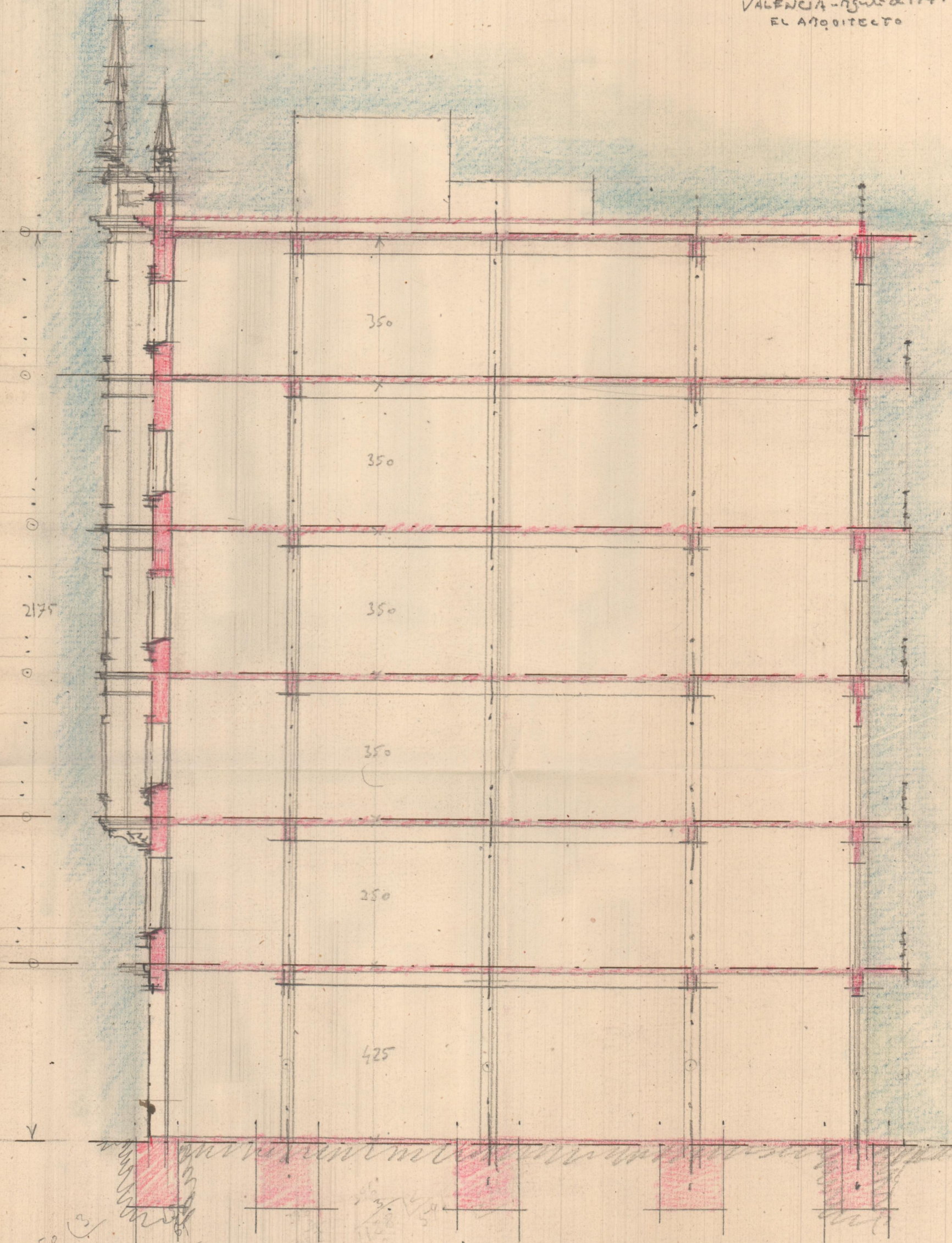
SECCION AB
