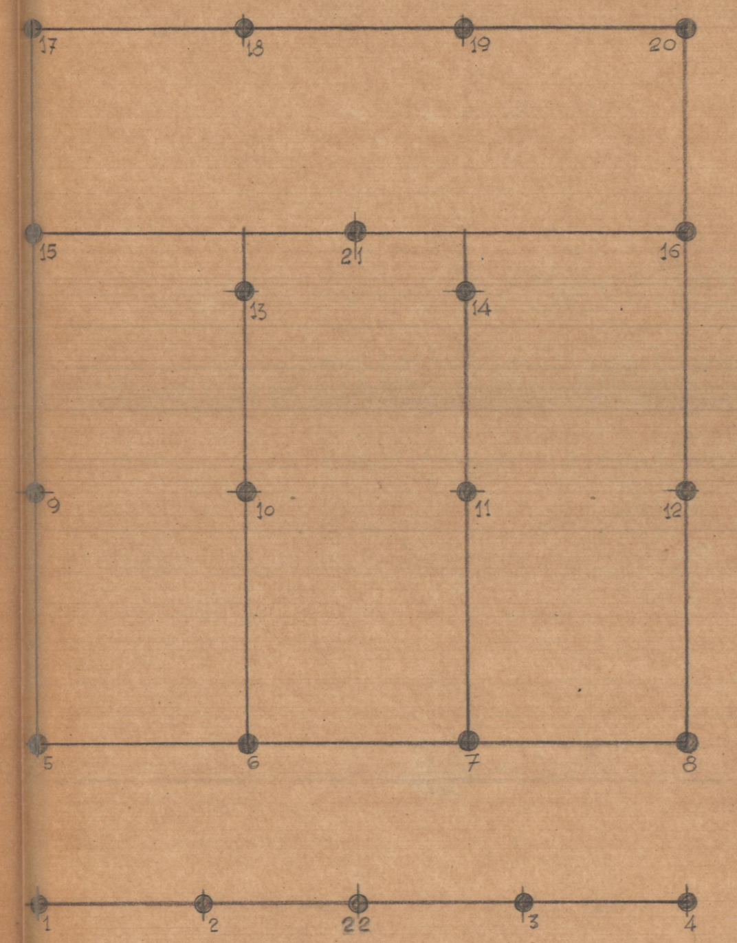
Pilares y entramado planta baja y pilas
