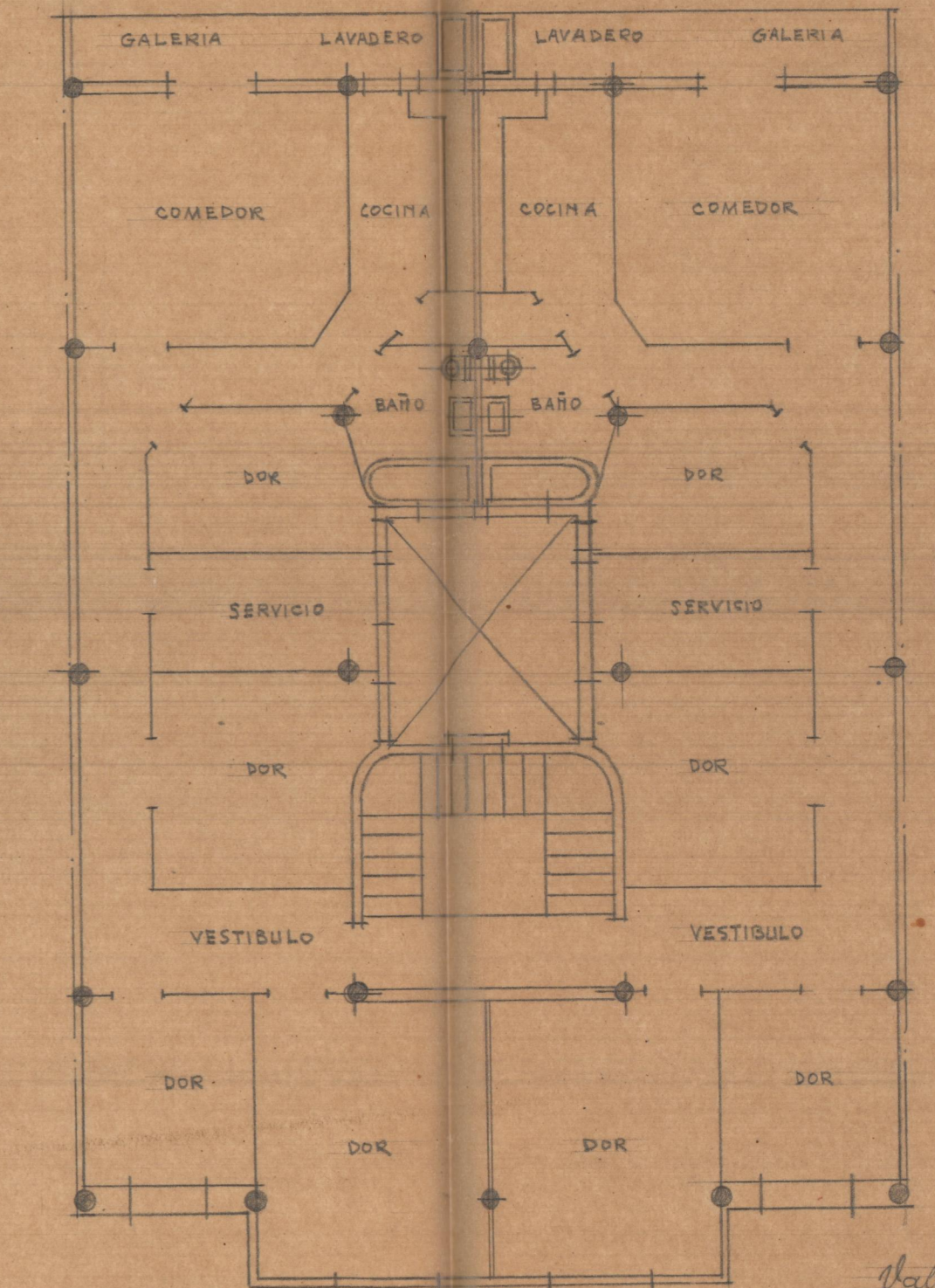
Planta pilas
