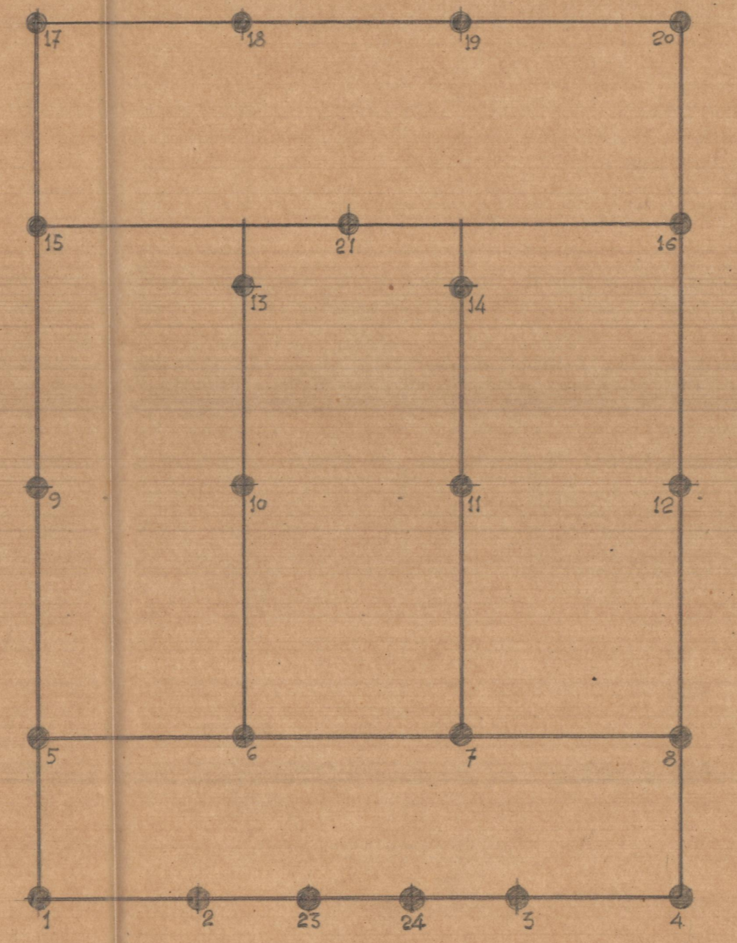
Pilares planta baja y entablado 2ª planta
