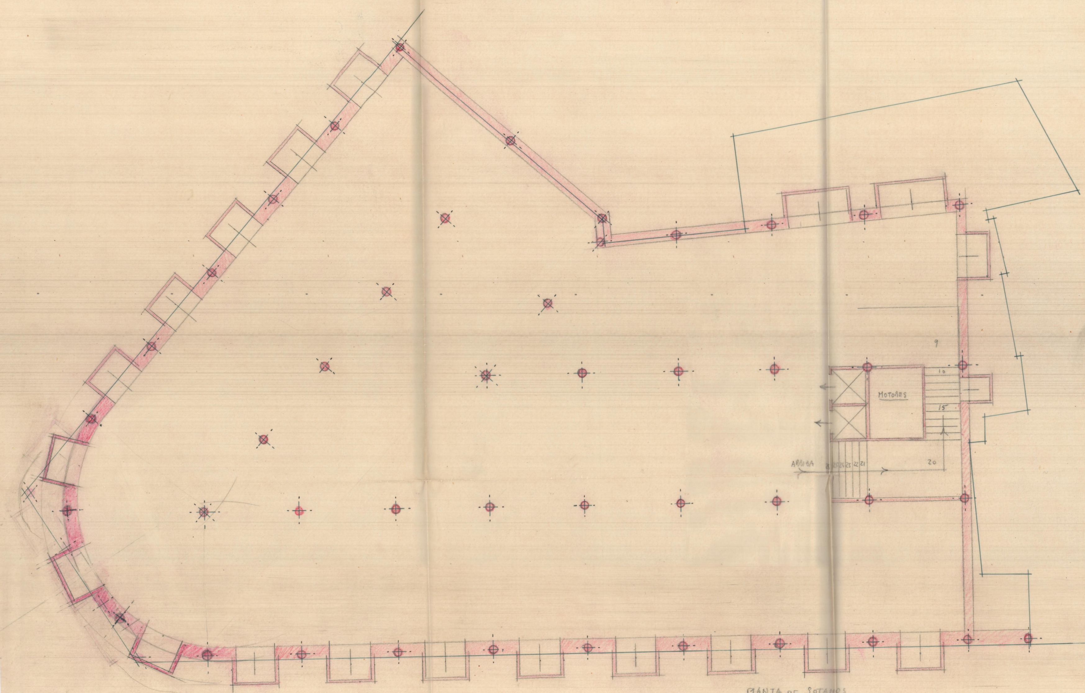
PLANTA DE SOTANOS E. 1:100
