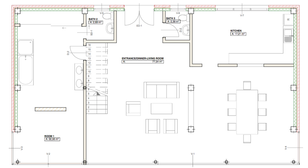
PLANTA SEGUNDA
