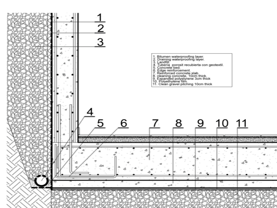
SECCION TRANSVERSAL
