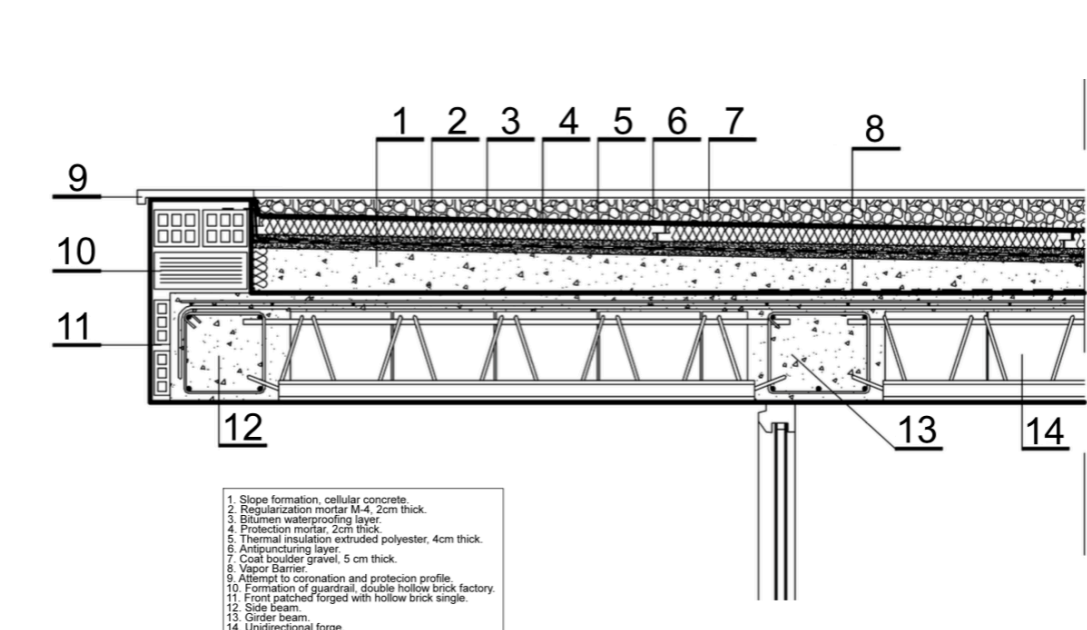
DETALLE CUBIERTA PLANA
