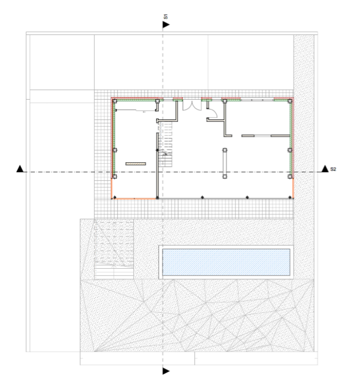
PLANTA CIMENTACION
