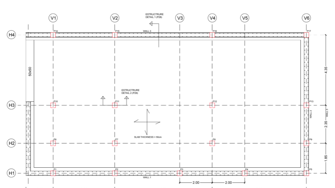
PLANO FORJADO - PLANTA SOTANO
