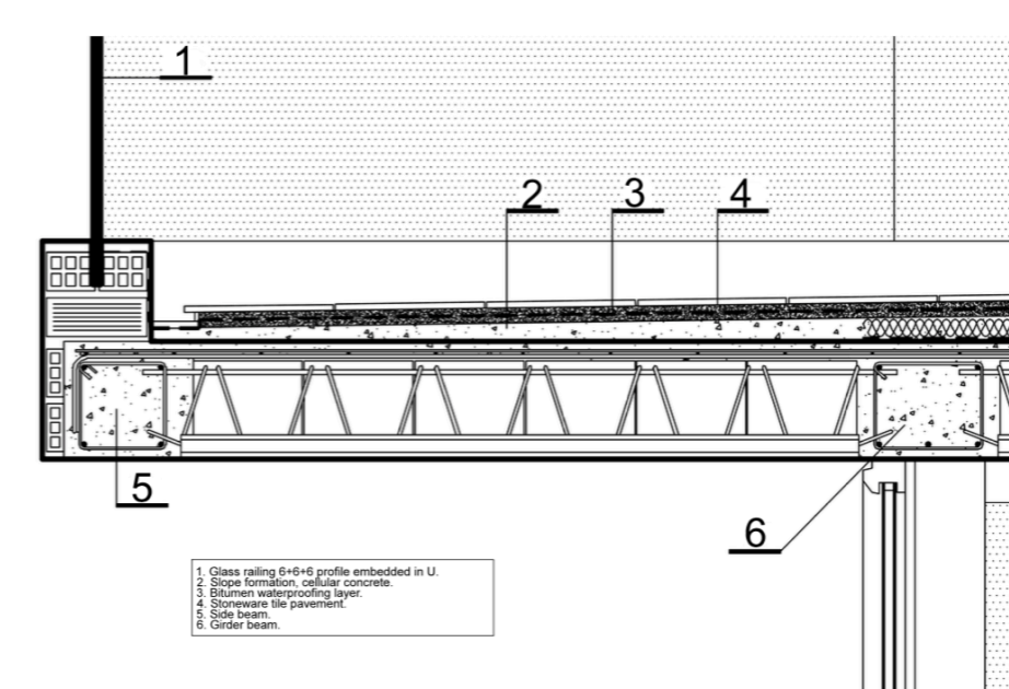
SECCION TRANSVERSAL
