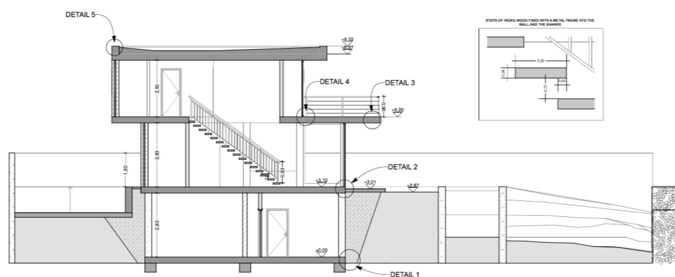
SECCION TRANSVERSAL
