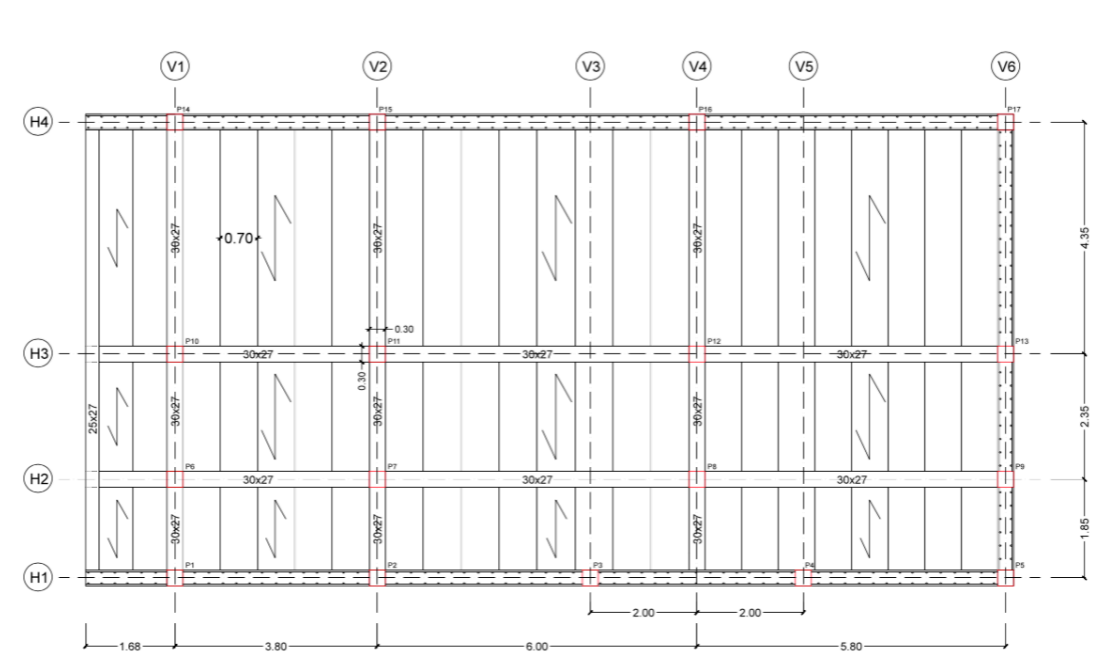
PLANO FORJADO - PLANTA SOTANO
