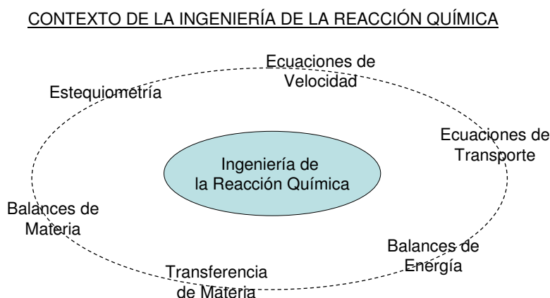
Figura 1.1: dentro del contexto de la Ingeniería de la Reacción Química es necesario hacer uso de conceptos derivados de áreas como la Termodinámica, la Cinética Química y de las ecuaciones de conservación de materia y energía.
