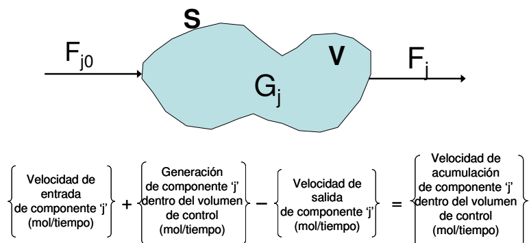
Figura 1.3: diagrama de la superficie y volumen de control de un sistema. Las ecuaciones de conservación de materia establecen la cantidad de materia que entra, sale y se transforma en el interior del volumen de control.
