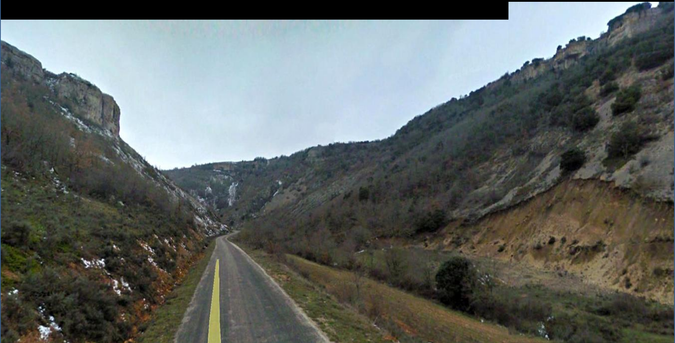
Margas y calizas arenosas del Cretácico Sup. N de San Andrés de Montearados, Burgos. SE Hoja de Polientes.
