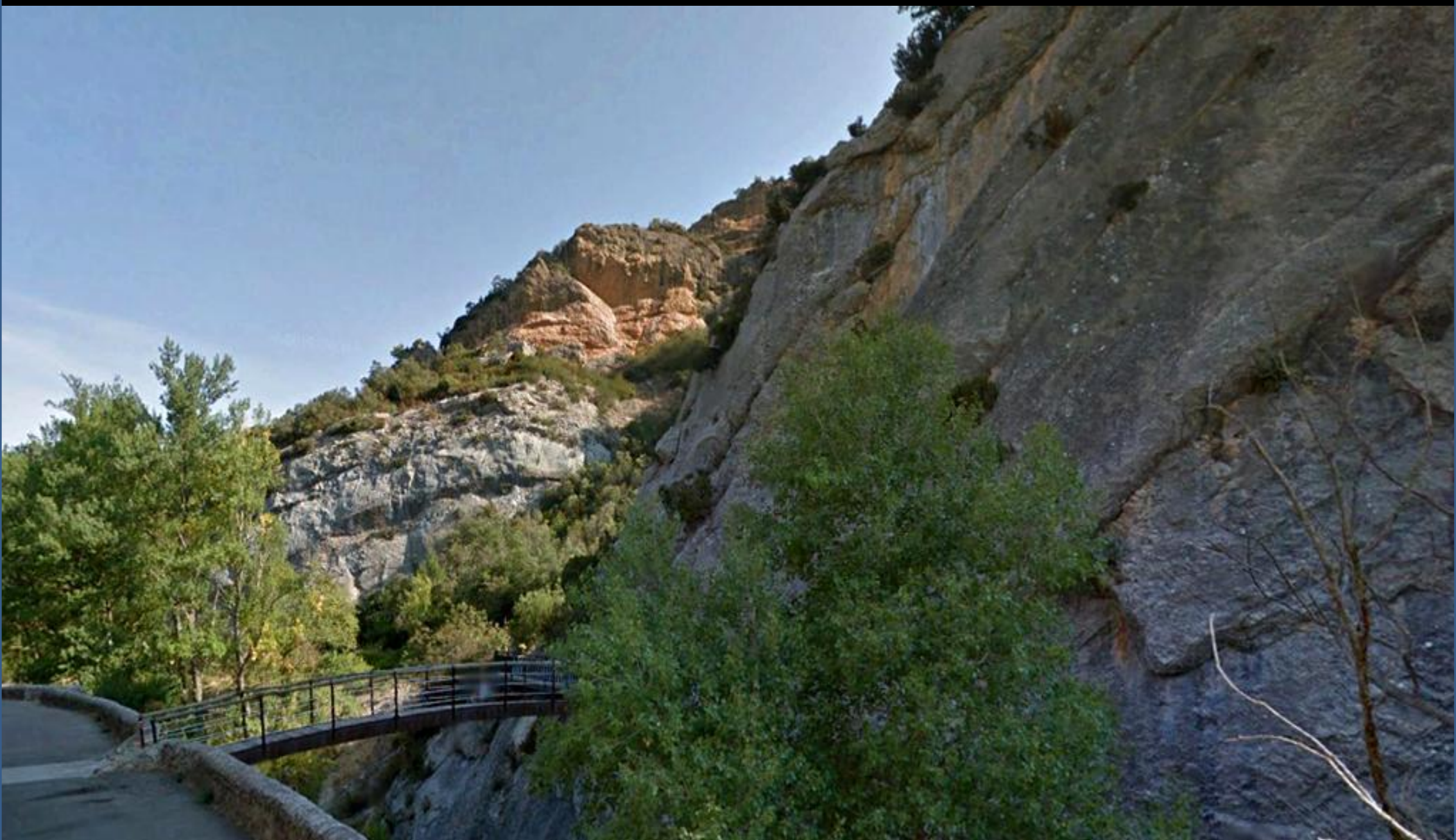
Calizas del Cretácico Sup. Desfiladero del Oca al N de Oña, Burgos. Centro W Hoja.
