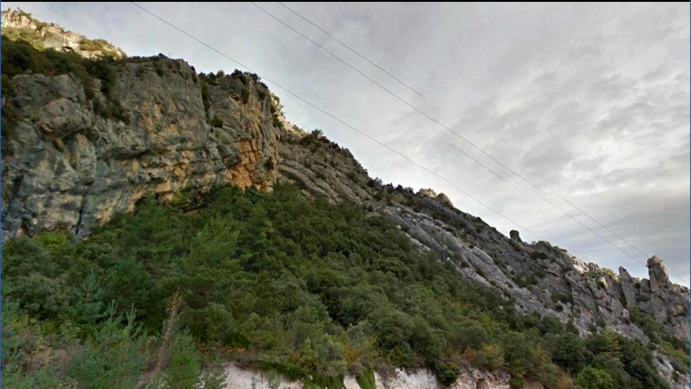
Antiforma en Mesozoicos. Barranco del Molinar, al NW de Ranera, Burgos. E Hoja de Oña.
