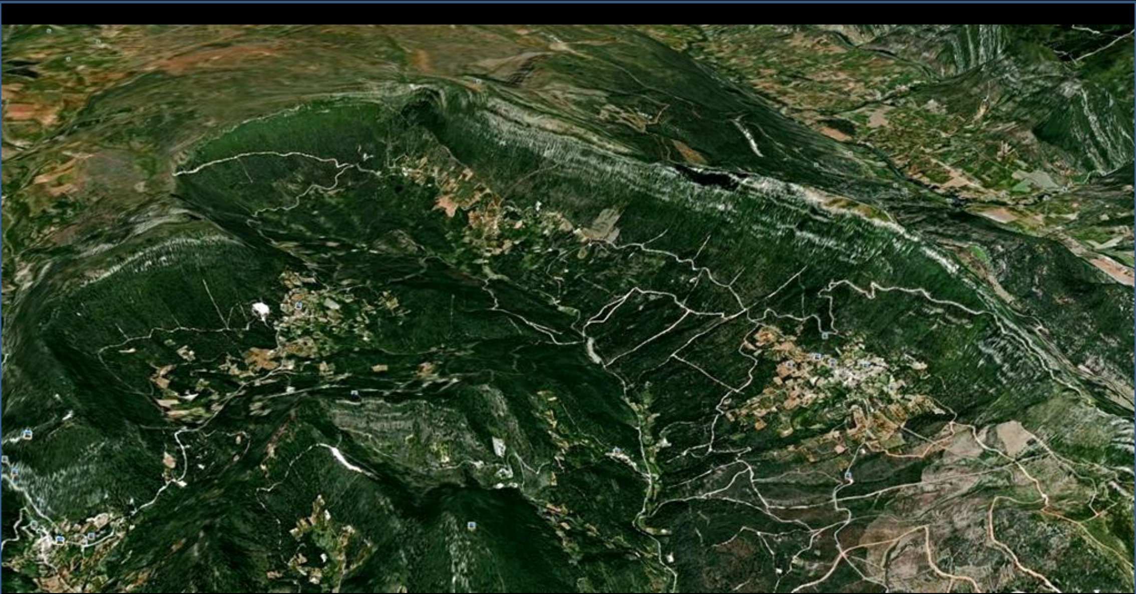
Perspectiva desde el ESE –relieve realzado- en la depresión de Rucandío. Wealdense rodeado de relieves calizos del Aptiense. E Hoja de Sedano.
