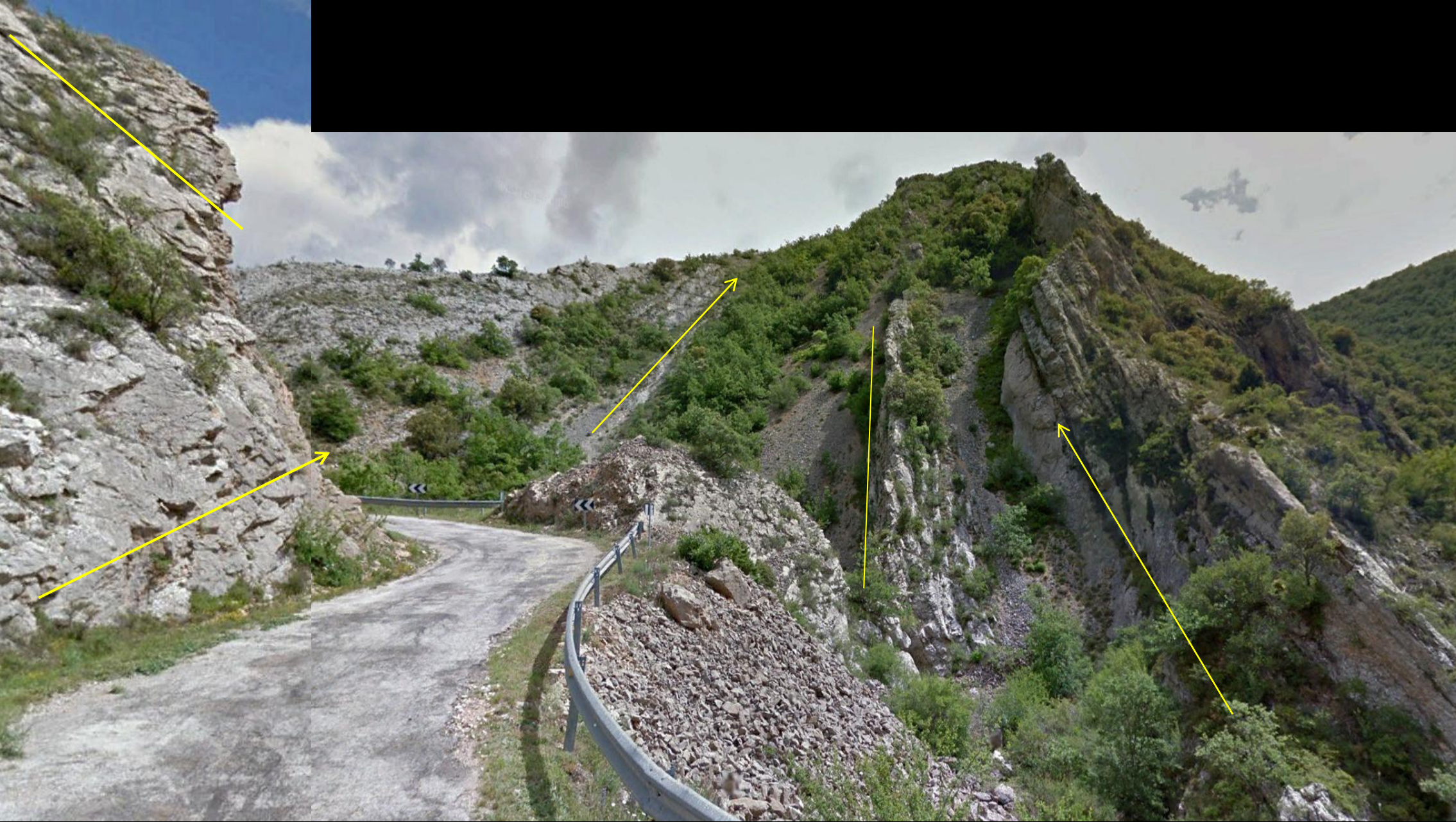
Zona de la anterior: Tectónica intensa en las calcarenitas del Santoniense, Cretácico Sup. N de Sedano hacia Nacedo, Burgos. Centro W Hoja.
