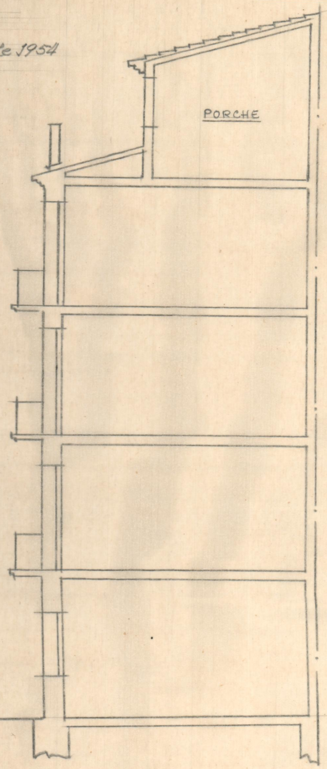
Sección transversal actual fol. A-B.
