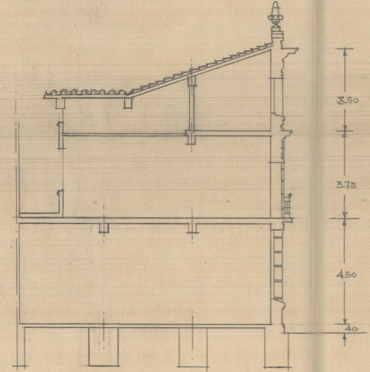
Sección por A.B.
