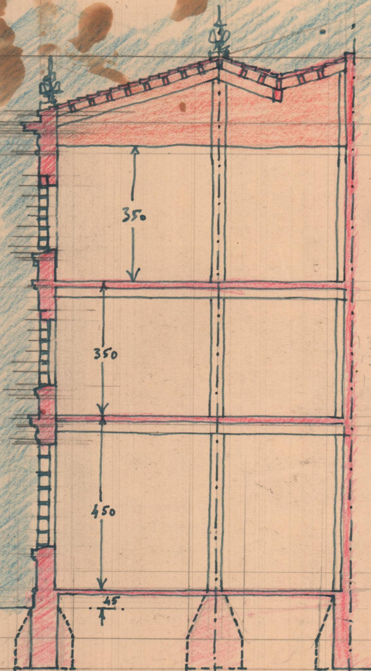
SECCION TRANSVERSAL
