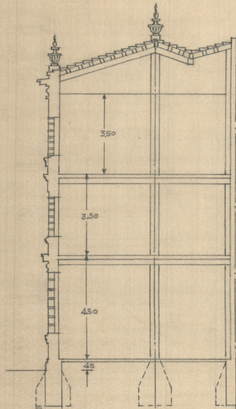
Sección transversal.
