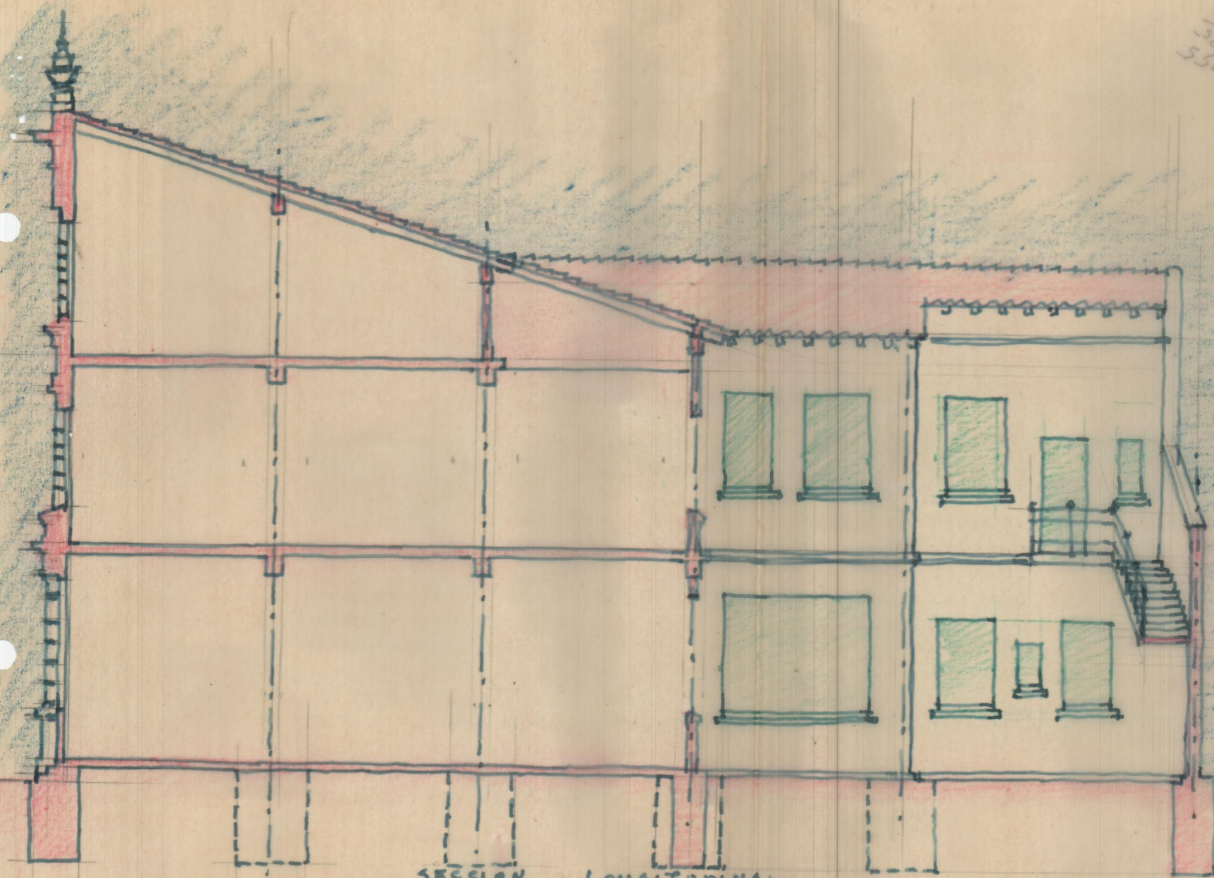
SECCION LONGITUDINAL
