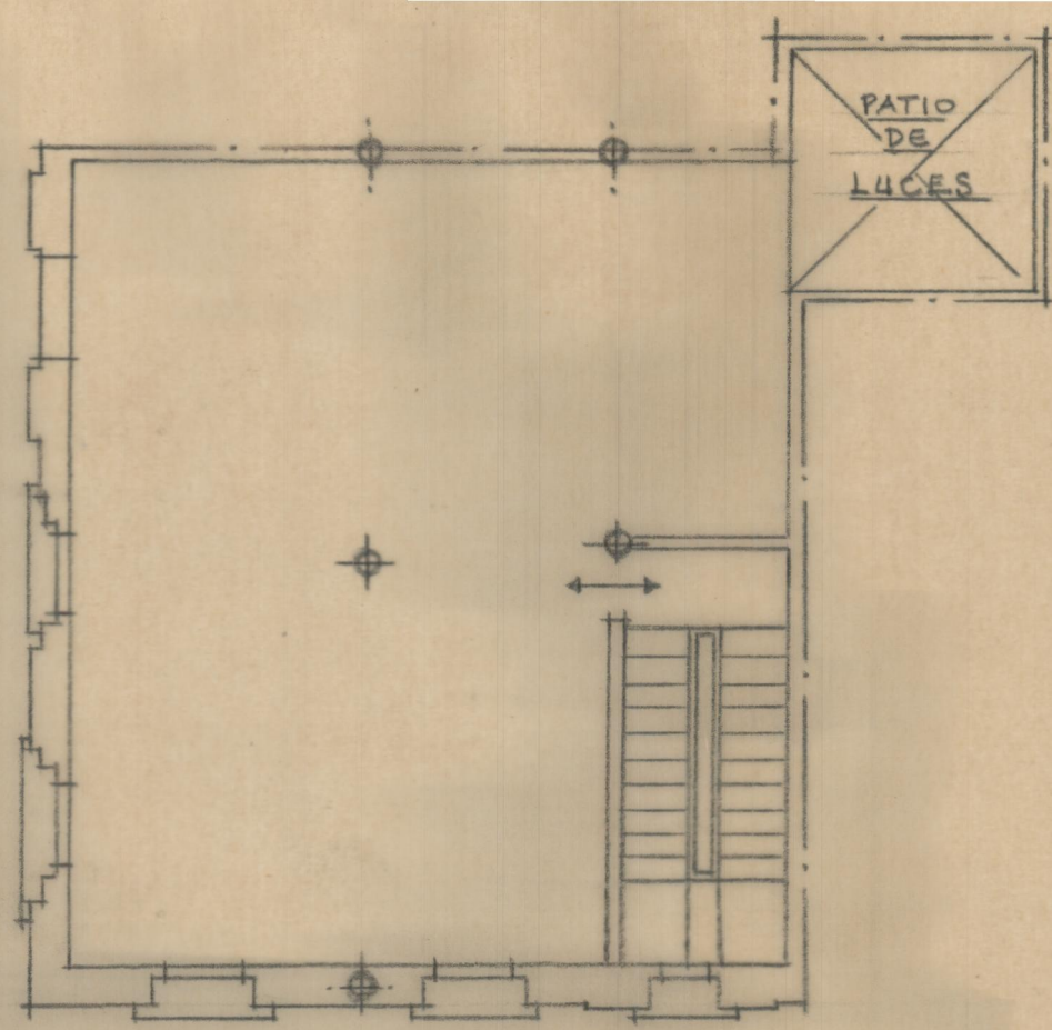
Ultima planta
