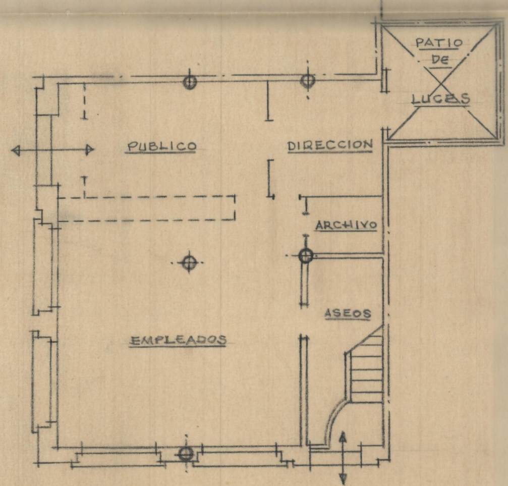
Planta baja
