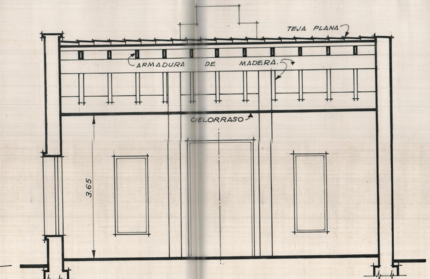
SECCIÓN A-B.
